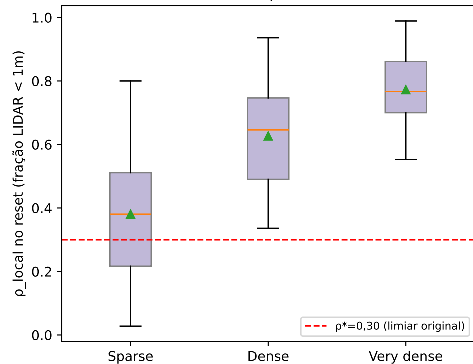
(c) Distribuição de \rho_{\text{local}} por mundo (500 trials, pool misto)
