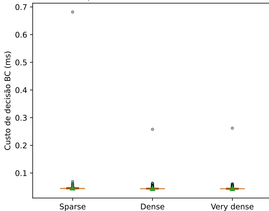
(b) Custo BC real — n=300/mundo praticamente sem variância
