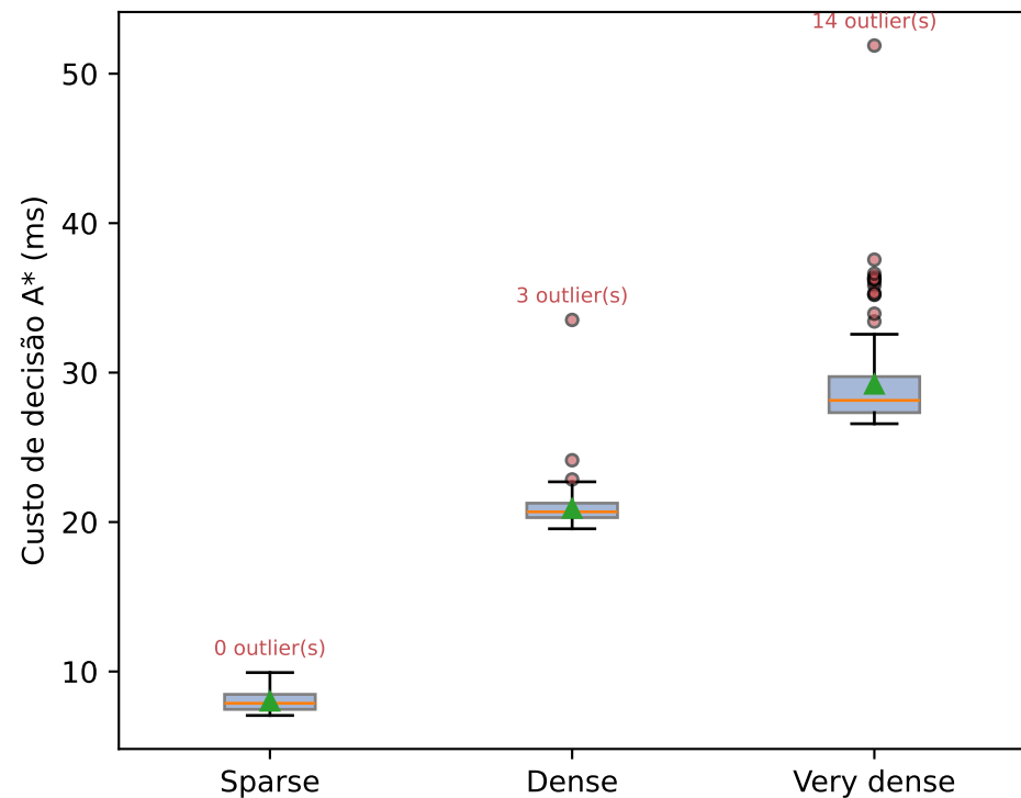
(a) Custo A* real — n=150/mundo círculos = outliers
