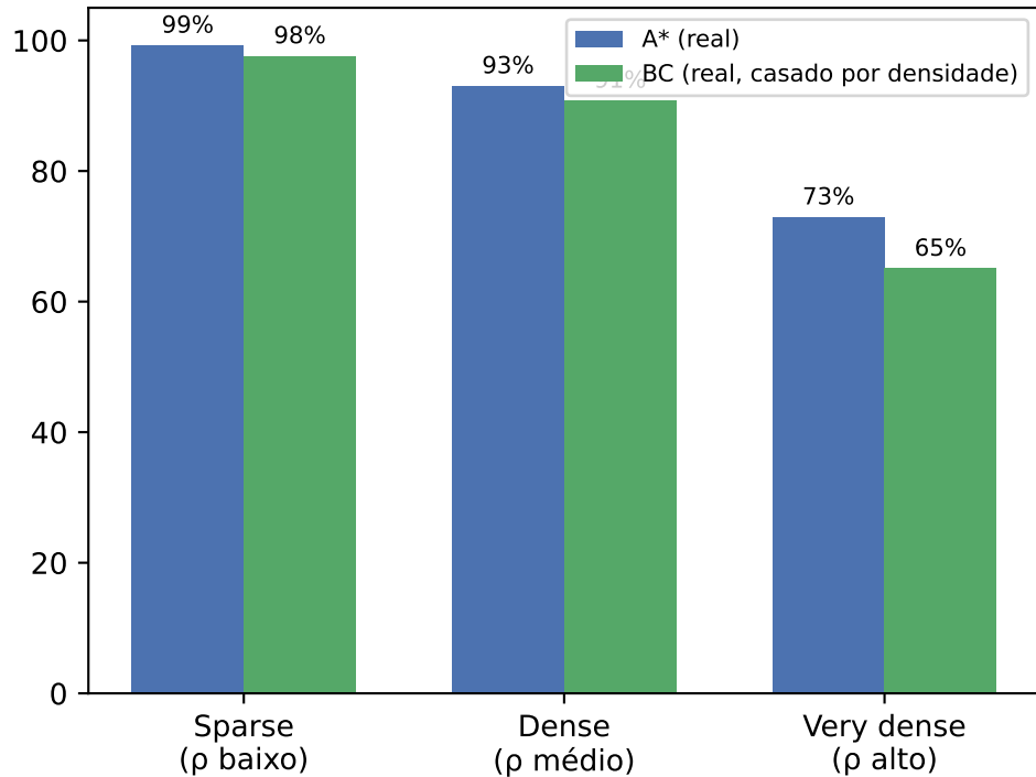
(a) Sucesso — A* real permanece à frente em todo regime
