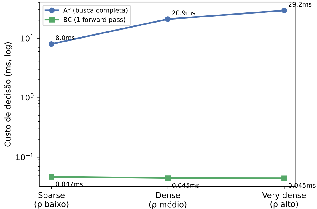
(b) Custo — BC ~656x mais barato em very_dense
