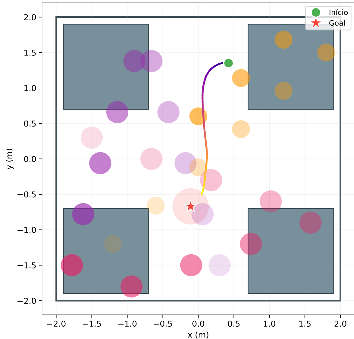
Trajetória p-criterion (BC) -- urban_grid, 3 obstáculo(s) dinâmico(s) 54 passos | ✓ Goal
