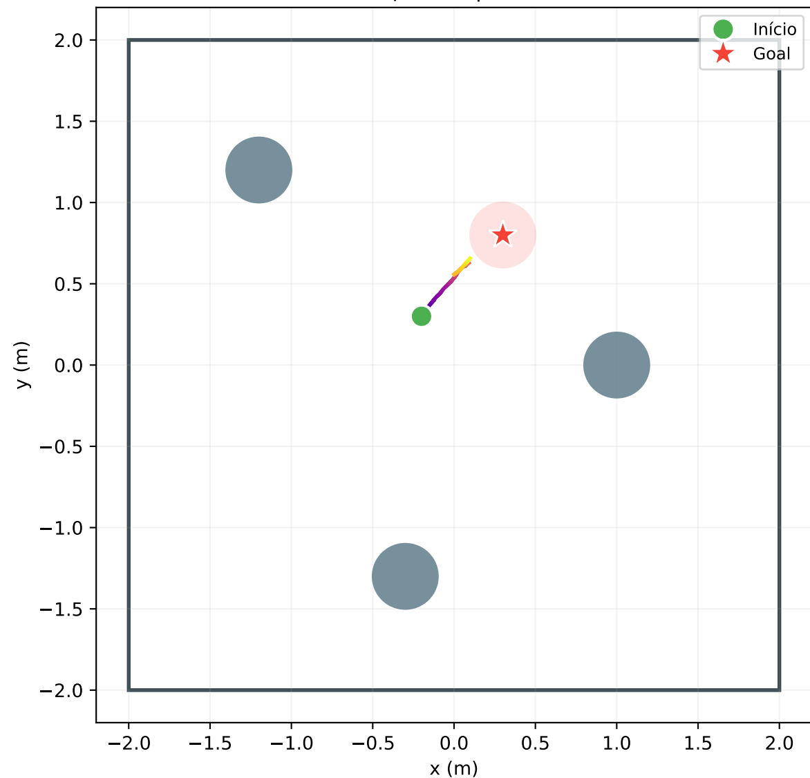
Trajetória SAC no Gazebo Classic real (sparse.world) 139 passos | ✓ Goal
