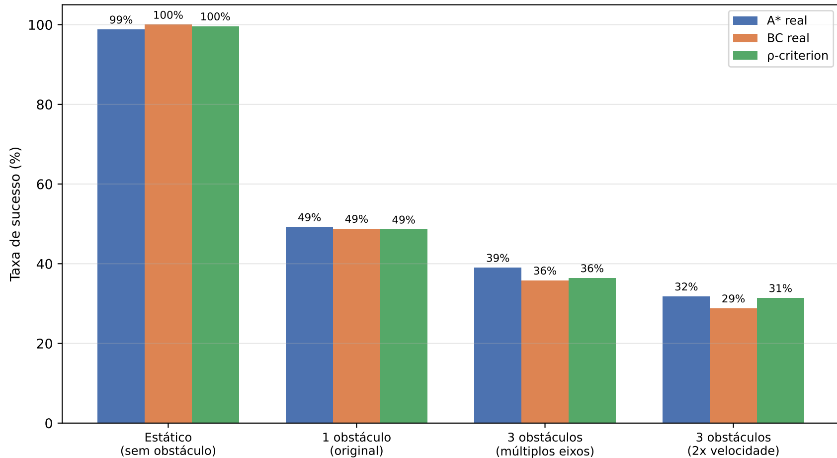
Cenário urbano: degradação de sucesso com número e velocidade de obstáculos dinâmicos (n=500 trials/condição, dados reais)
