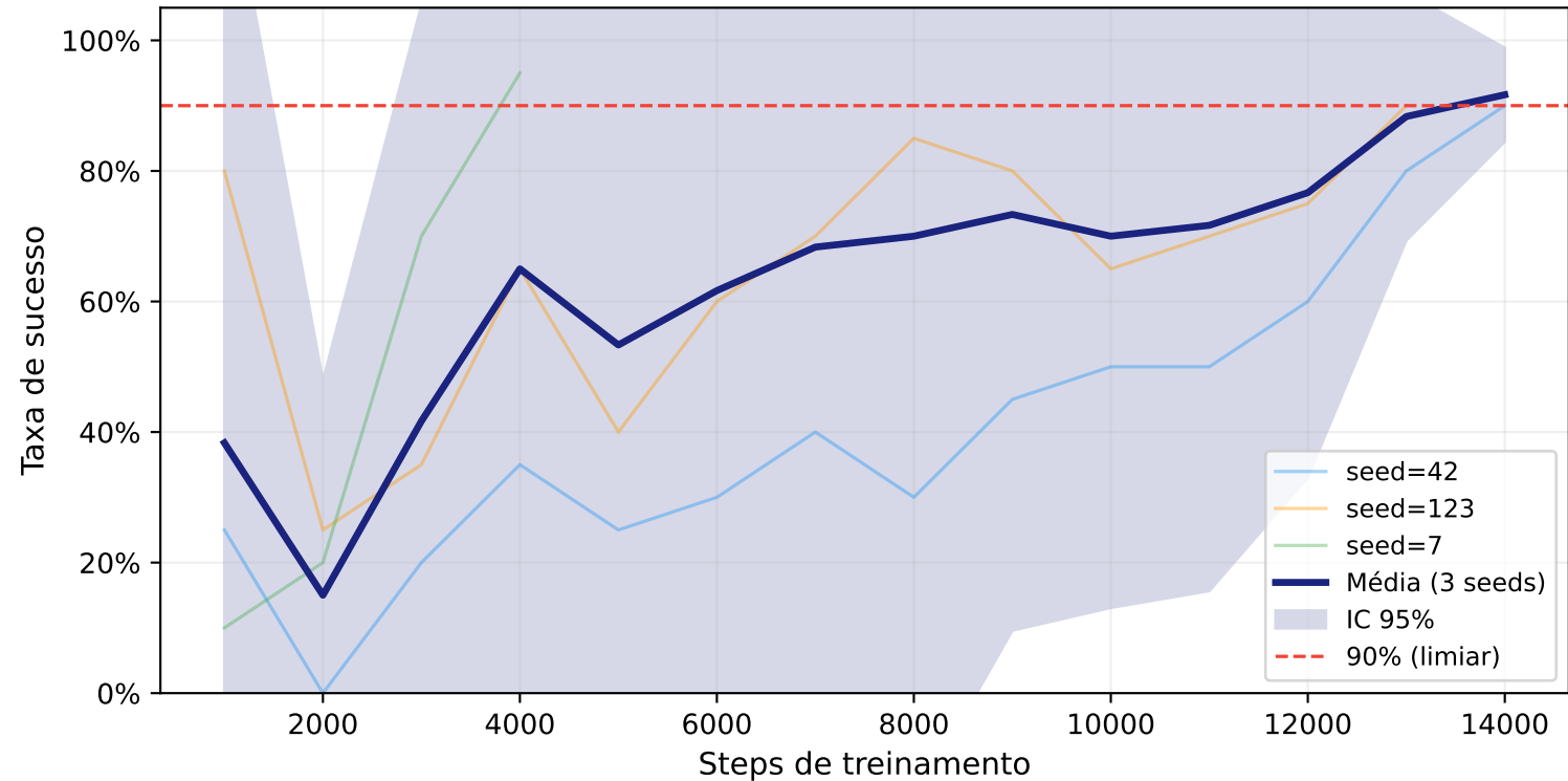
Curva de Aprendizagem SAC — Env 2D (3 seeds independentes) world=sparse, MAX_STEPS=200, R_APPROACH=10
