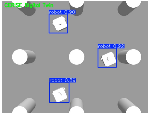
Figura 1. Vista aérea da câmera fixa sobre os três robôs TurtleBot3, com as caixas delimitadoras e a confiança de detecção do modelo YOLO sobrepostas em tempo real.
