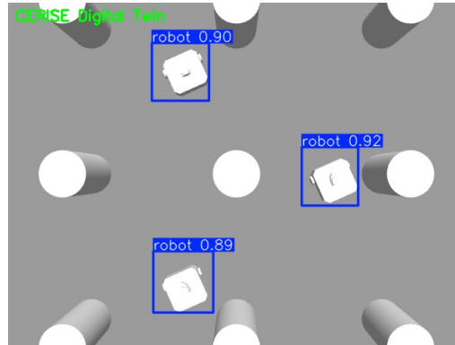
Figura 1. Vista aérea da câmera fixa sobre os três robôs TurtleBot3, com as caixas delimitadoras e a confiança de detecção do modelo YOLO sobrepostas em tempo real.
