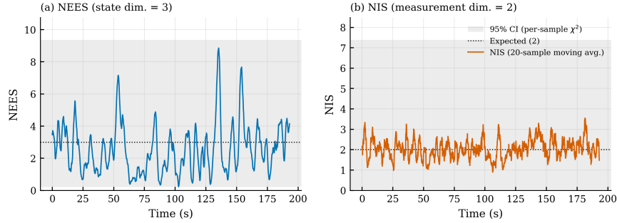
Figura 2. Consistência de NEES e NIS ao longo da validação sintética de Monte Carlo (30 sementes, 2000 passos cada). Ambas as estatísticas acompanham seus valores teóricos esperados, indicando um filtro bem calibrado.
