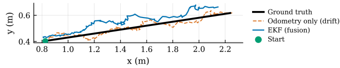
Figura 3. Trajetória estimada sob deriva agressiva, Cenário 2 (movimento reto). O EKF (azul) acompanha a ground truth (preto) mais de perto que a odometria bruta com deriva (laranja, tracejado).
