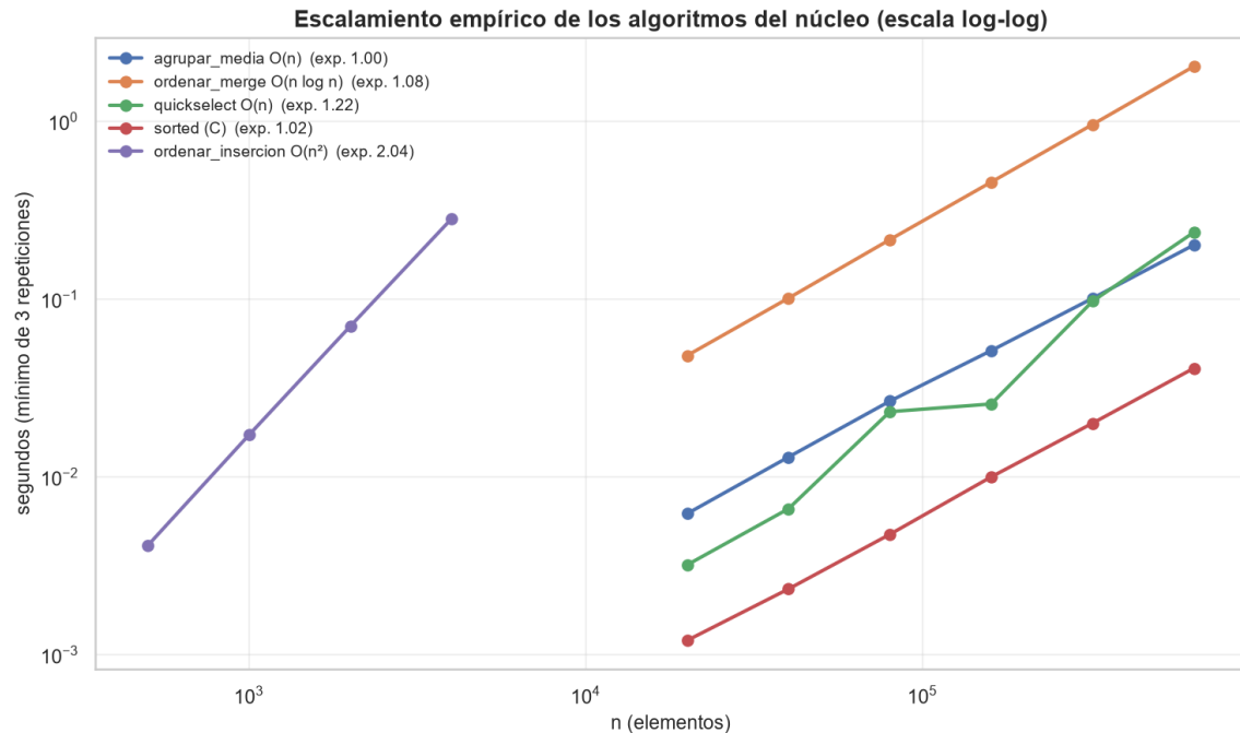
Figura 1. Escalamiento empírico de los algoritmos del núcleo en escala log-log; la pendiente de cada recta es el exponente de crecimiento.
