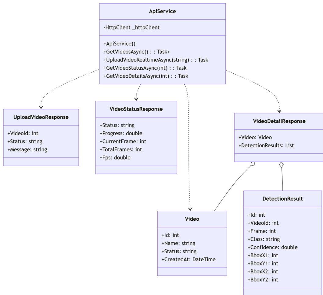
图 4-8ApiService模块
