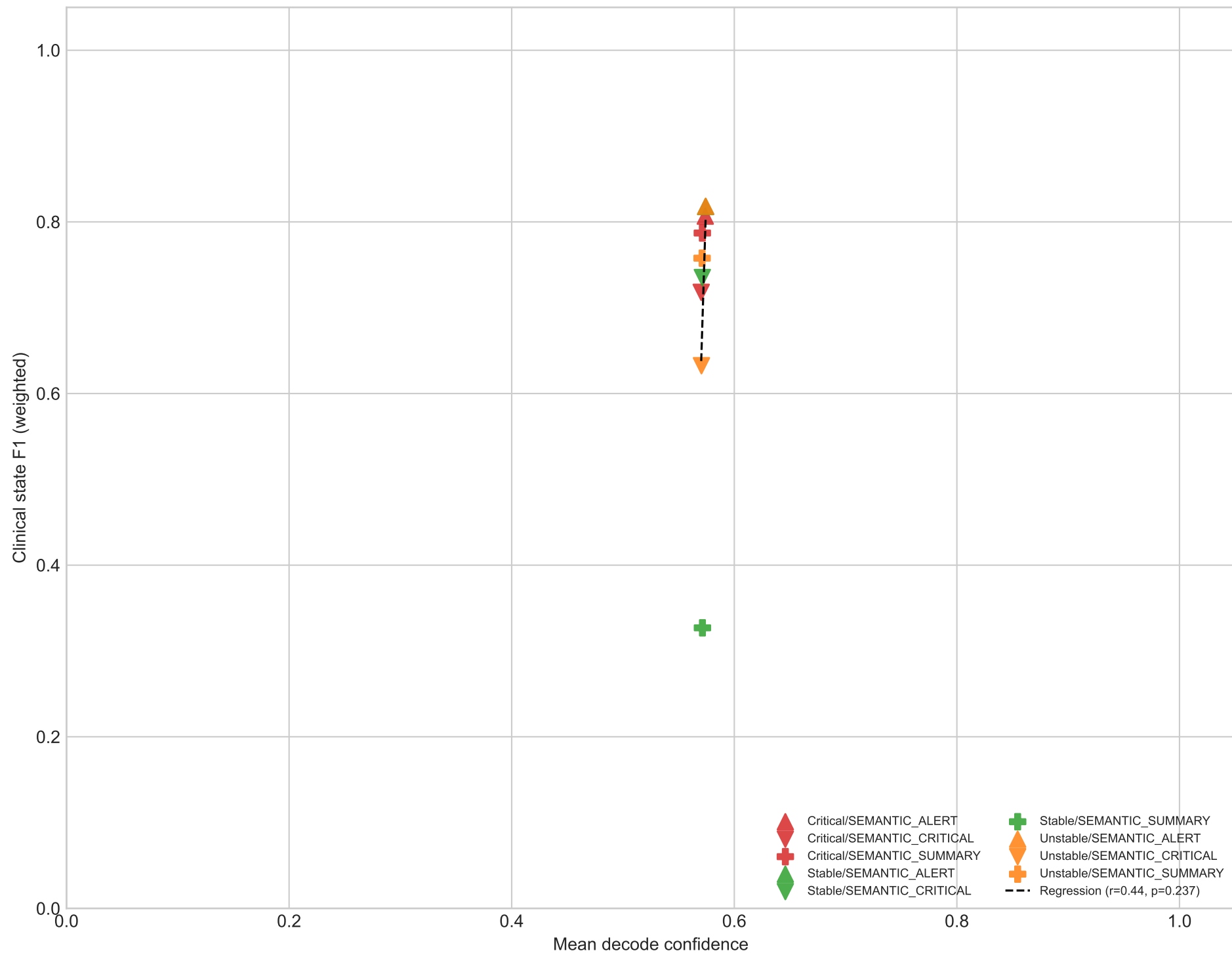
Decode confidence vs clinical state F1
