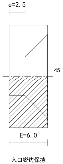
孔口局部 3:1
