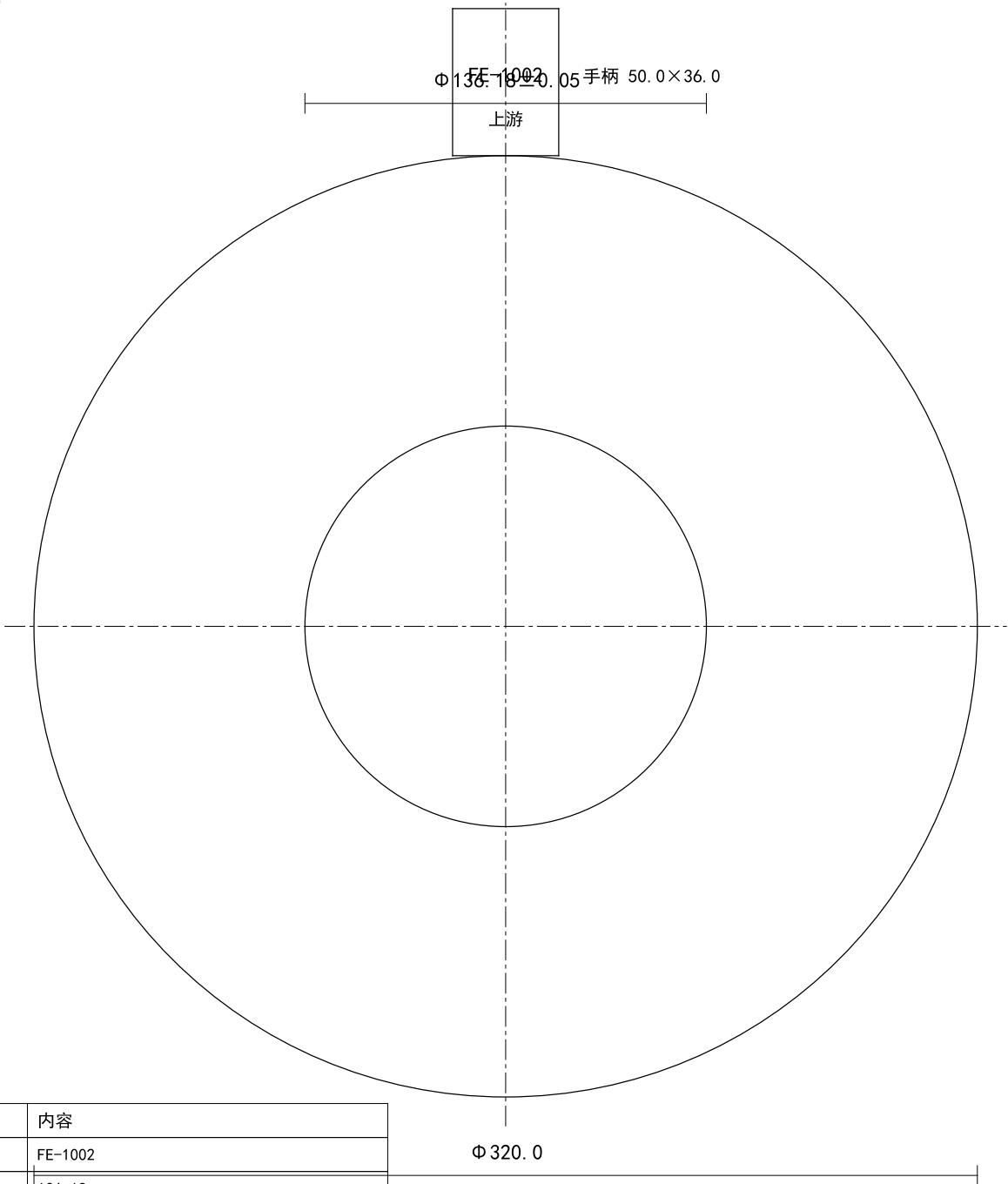
主视（上游面）比例1:2
