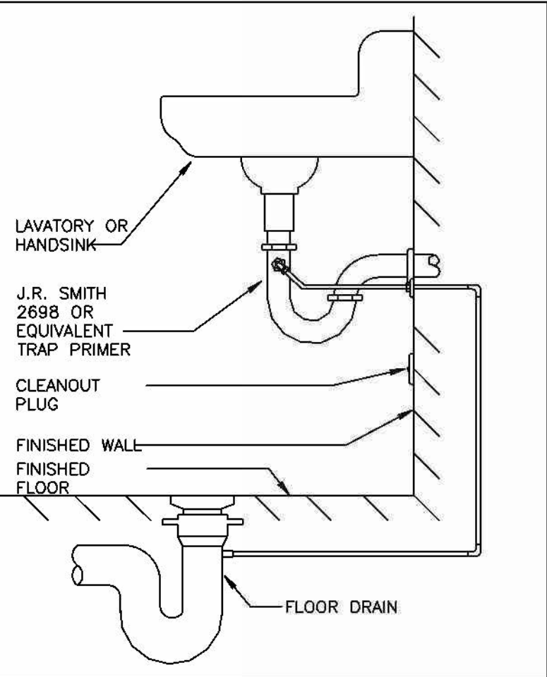
TRAP PRIMER DETAIL
