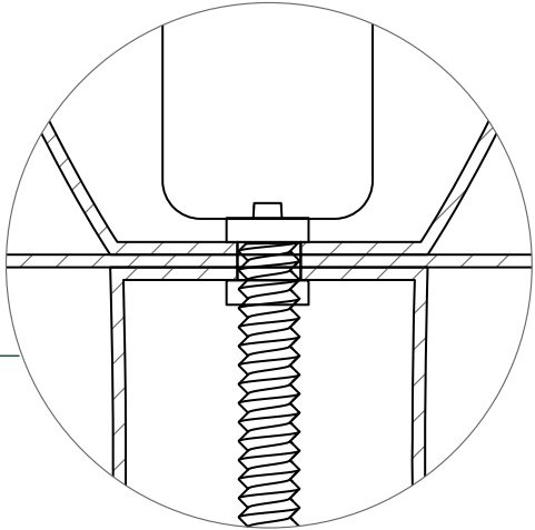
DETALLE B
