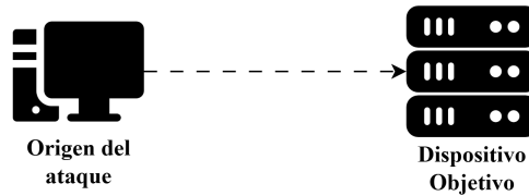
Figura 3.4: Ataque DoS
