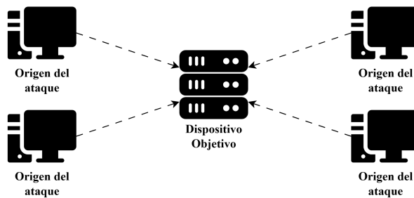
Figura 3.5: Ataque DDoS
