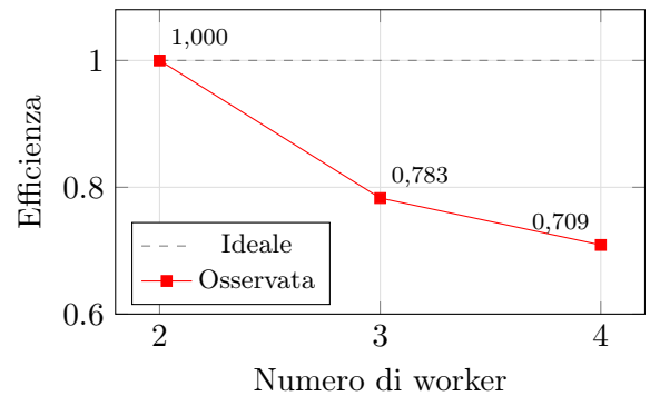
Figura 2: Analisi di strong scaling.
