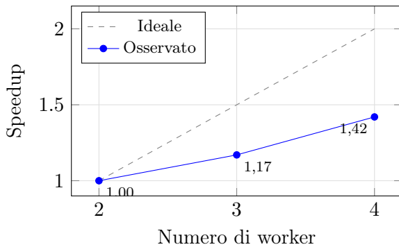
Figura 2: Analisi di strong scaling.
