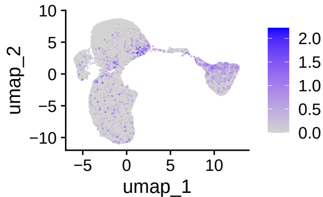
SPOCD1
