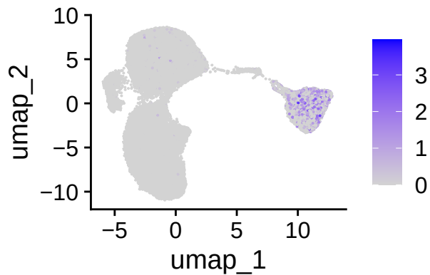
GPT
