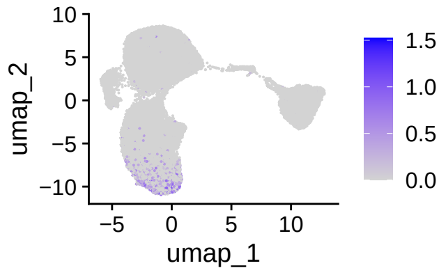
GPT
