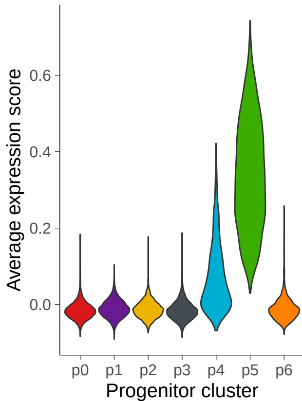
S.Score
