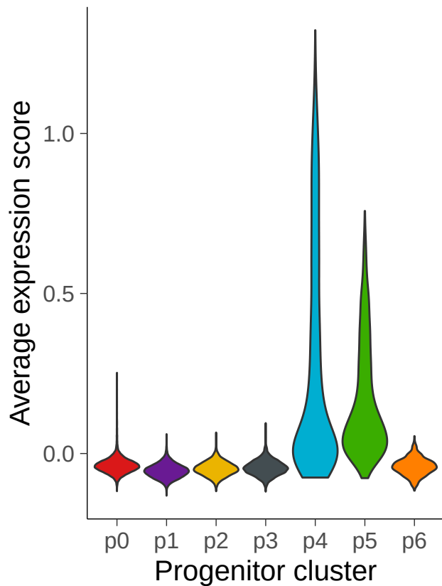
G2M.Score
