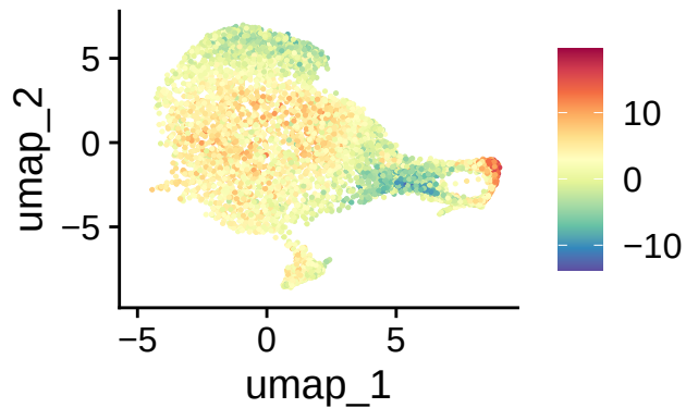
integratedrpca_4
