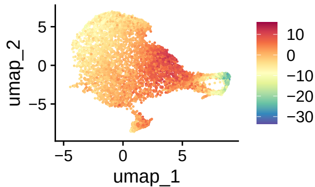
integratedrpca_3
