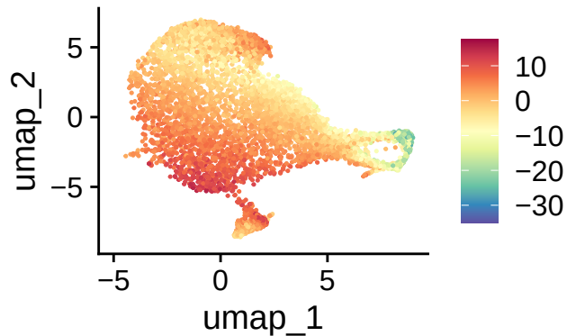
integratedrpca_4
