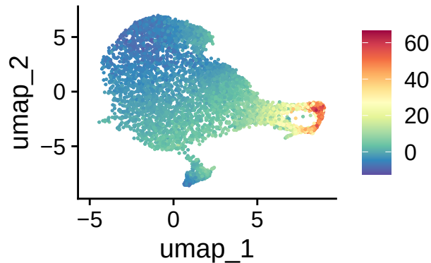
integratedrpca_3
