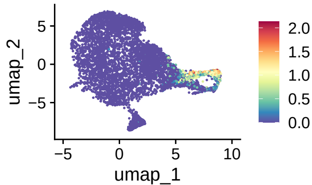
CLSPN
