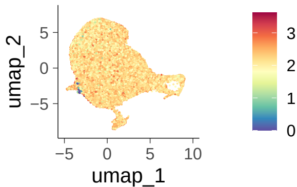
RPL27A
