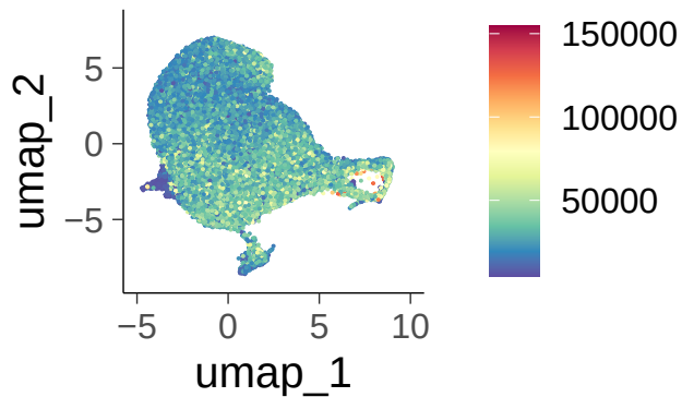
RPL27A
