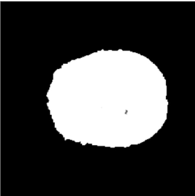
z = 4
