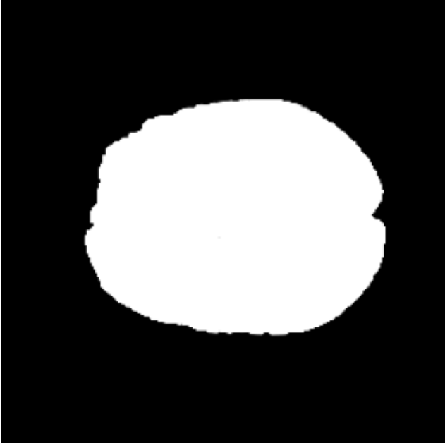
z = 4
