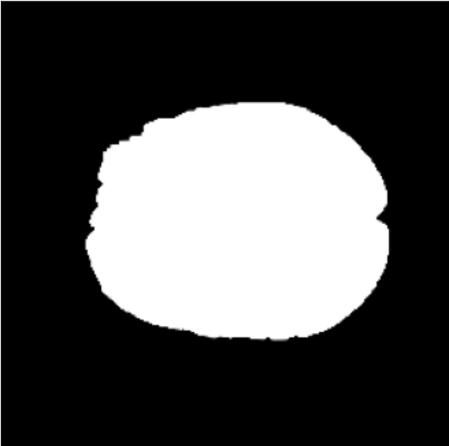
z = 2
