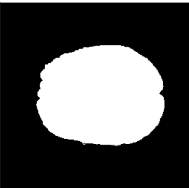
z = 7
