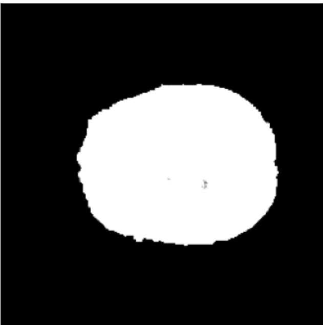
z = 5
