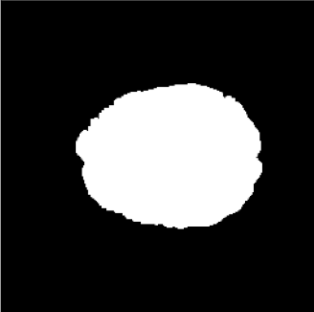
z = 5
