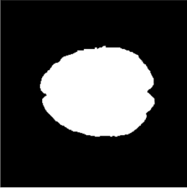
z = 1
