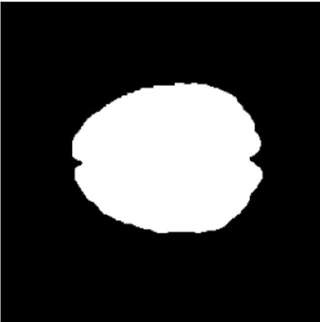
z = 3
