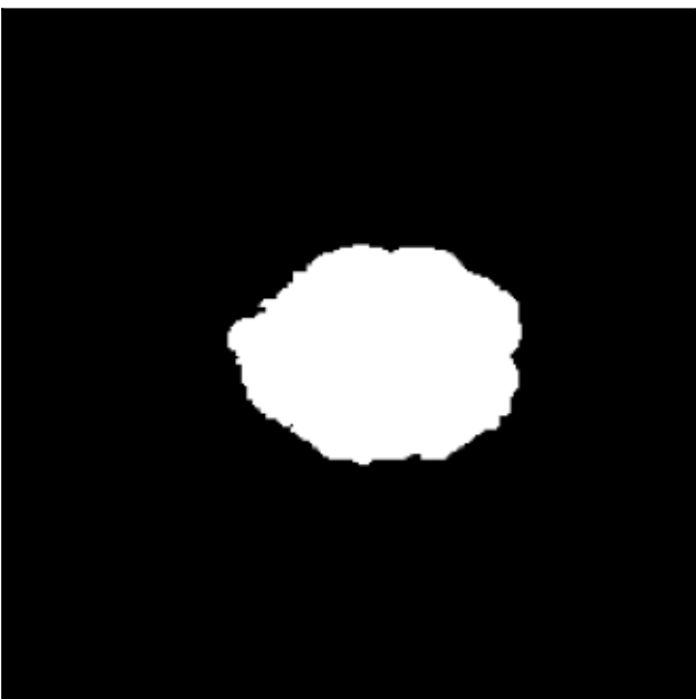
z = 2
