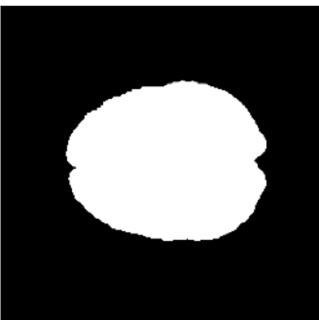
z = 5
