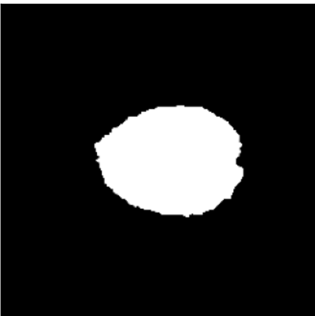
z = 6
