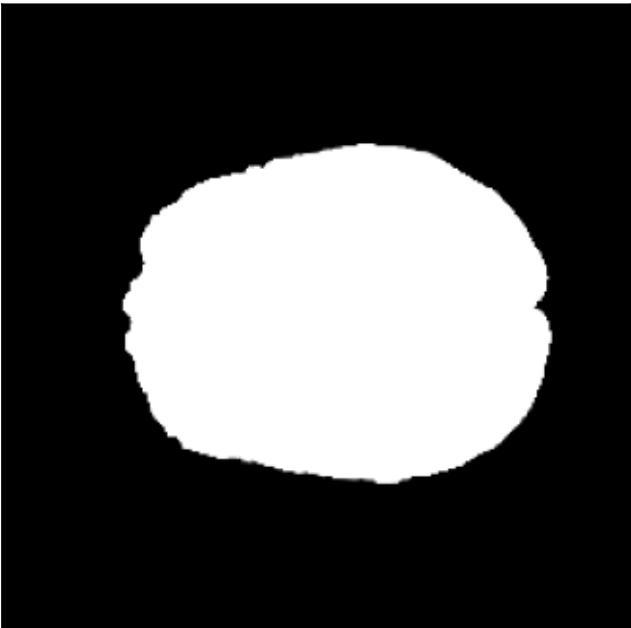
z = 3
