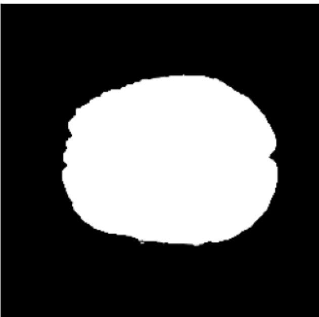
z = 6
