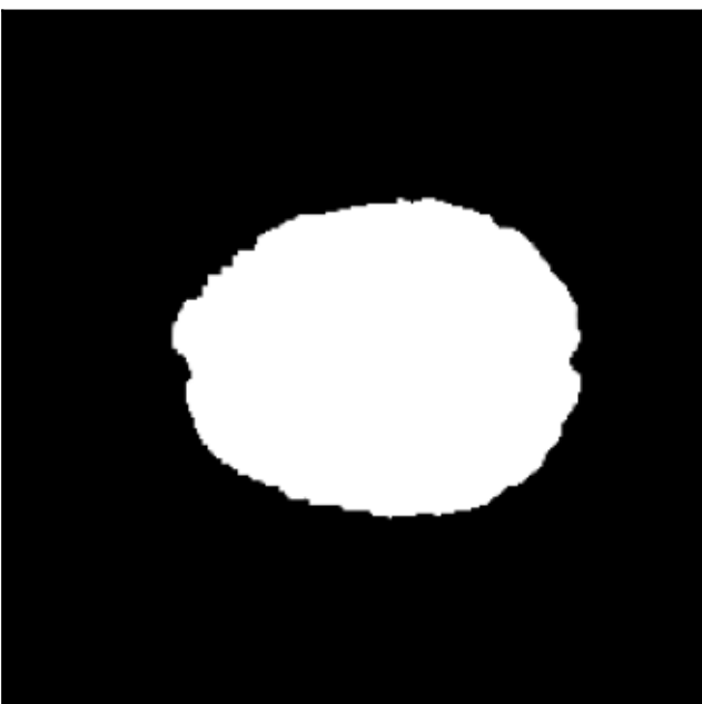
z = 7
