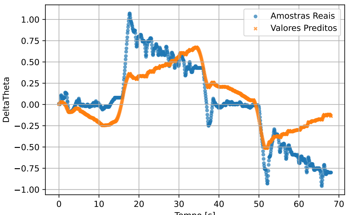
train1 - DeltaTheta
