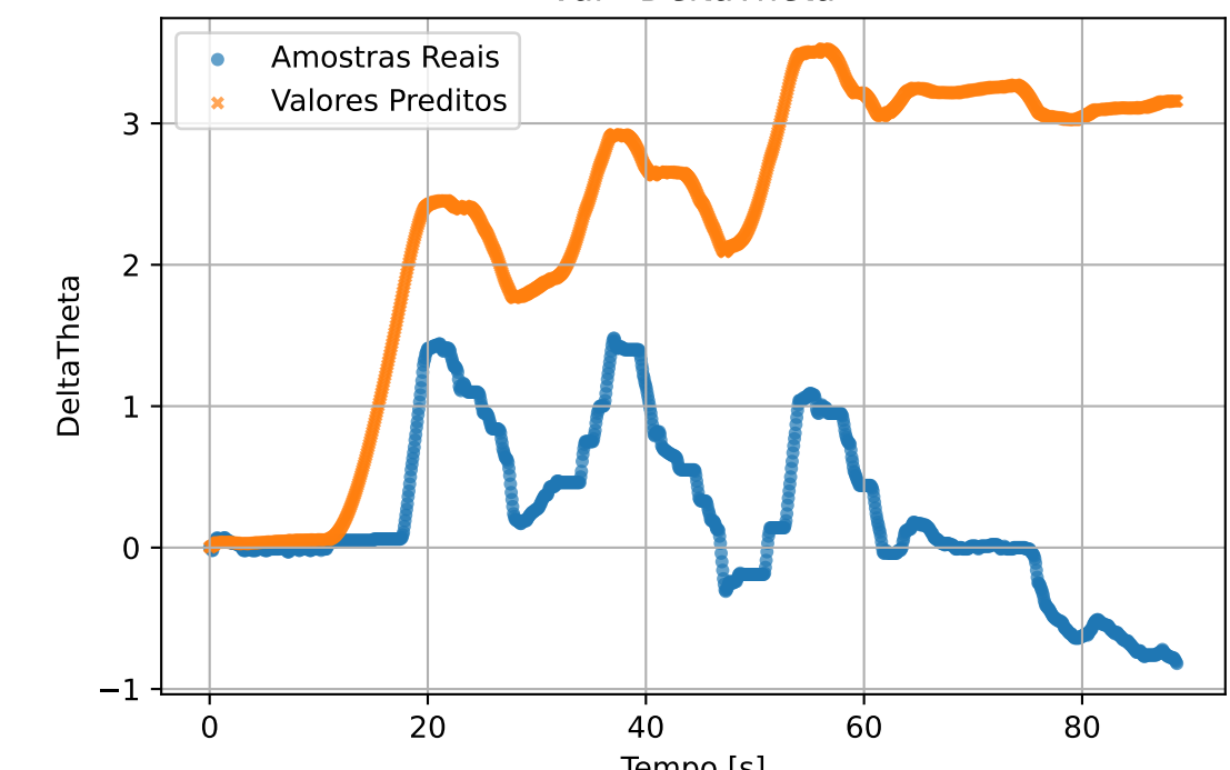
val - DeltaTheta
