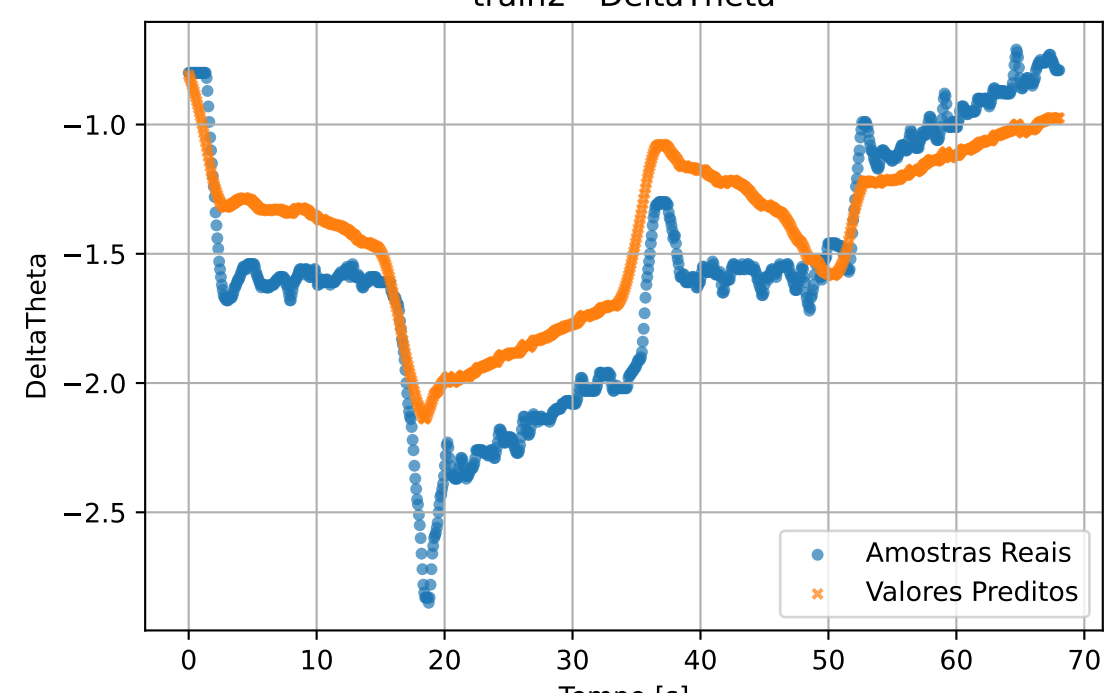
train2 - DeltaTheta
