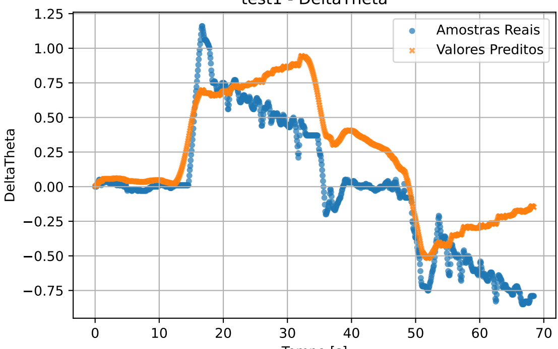
test1 - DeltaTheta
