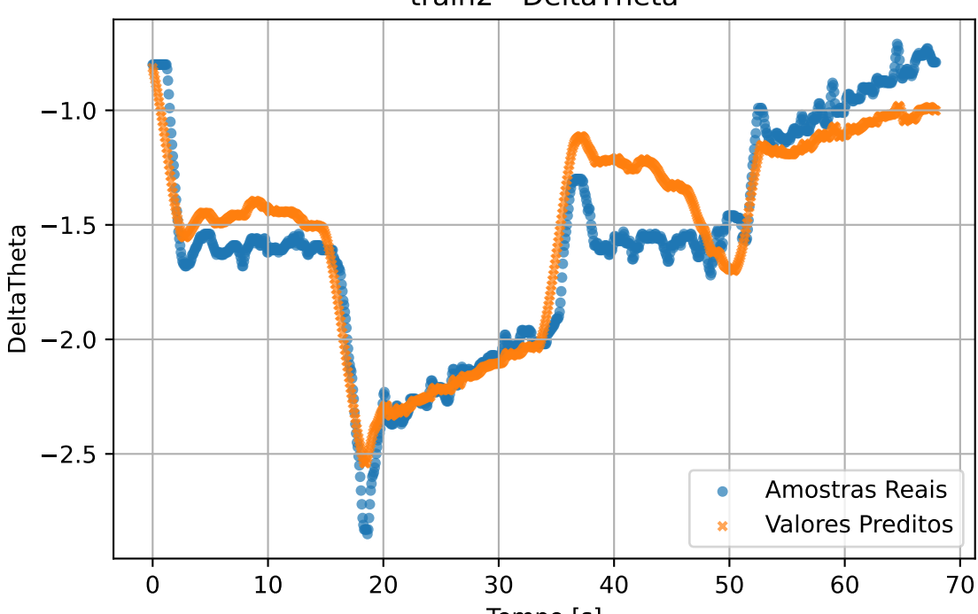
train2 - DeltaTheta
