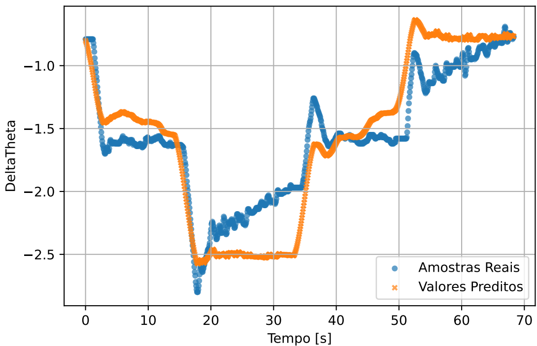
test3 - DeltaTheta
