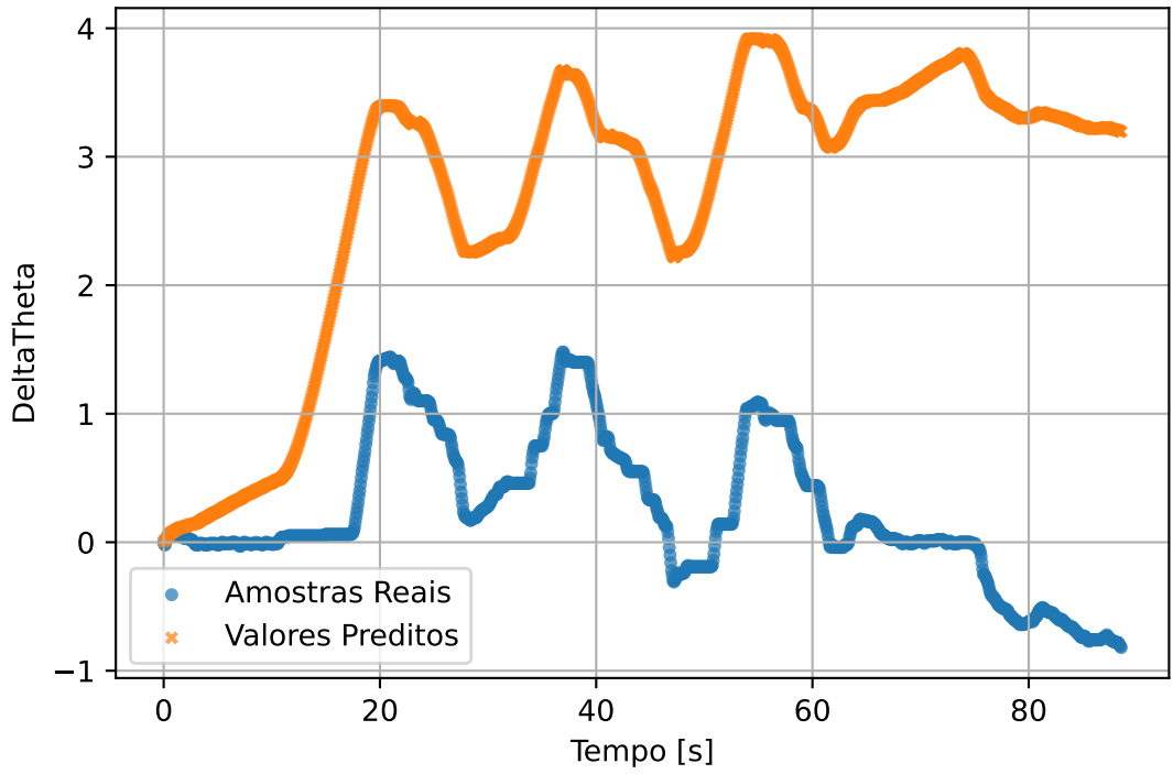
val - DeltaTheta
