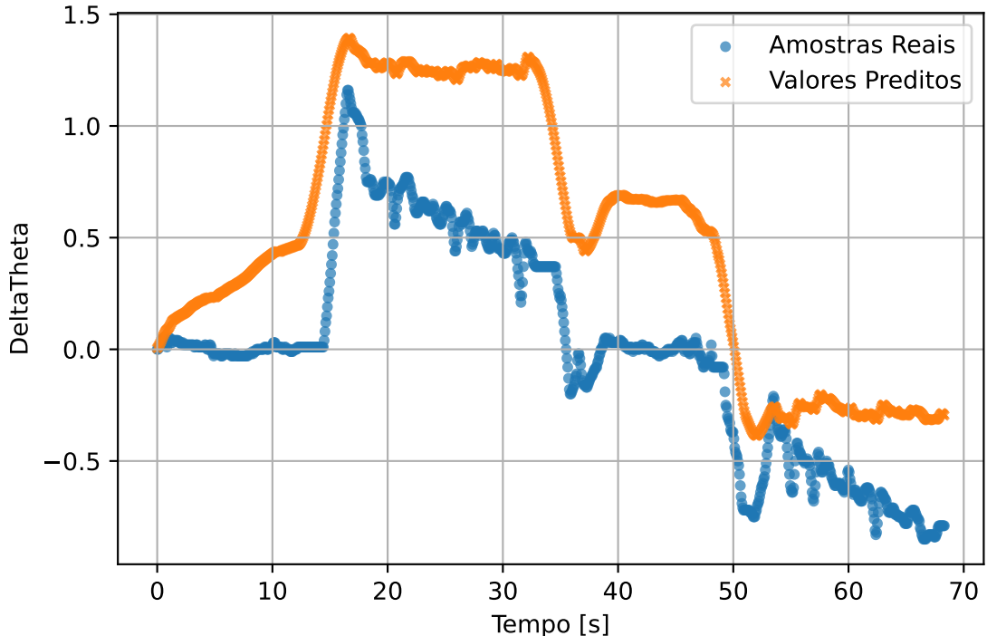
test2 - DeltaTheta
