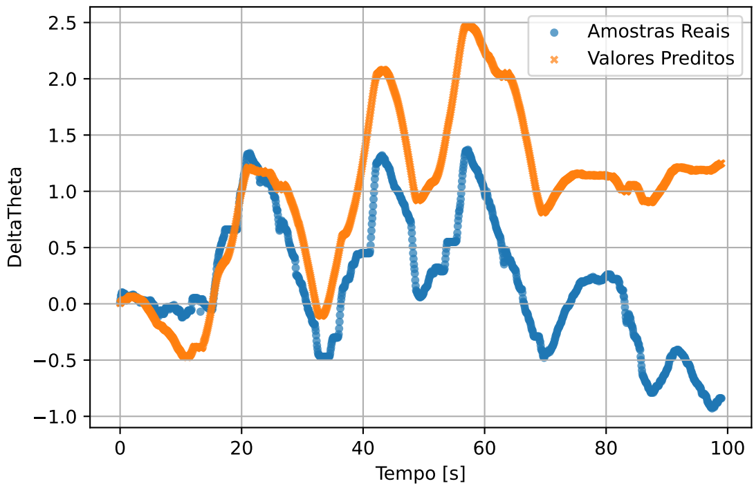
val - DeltaTheta
