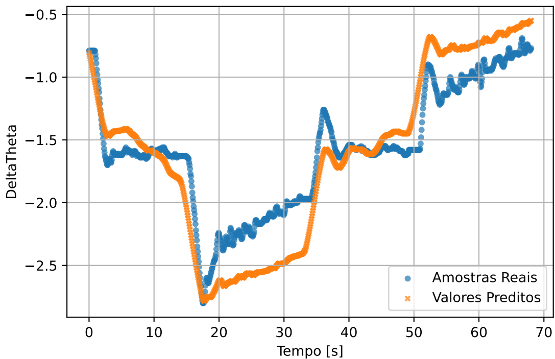
test3 - DeltaTheta
