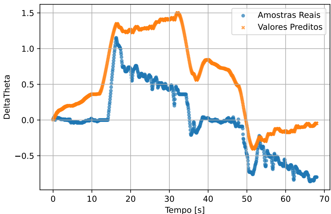
test2 - DeltaTheta
