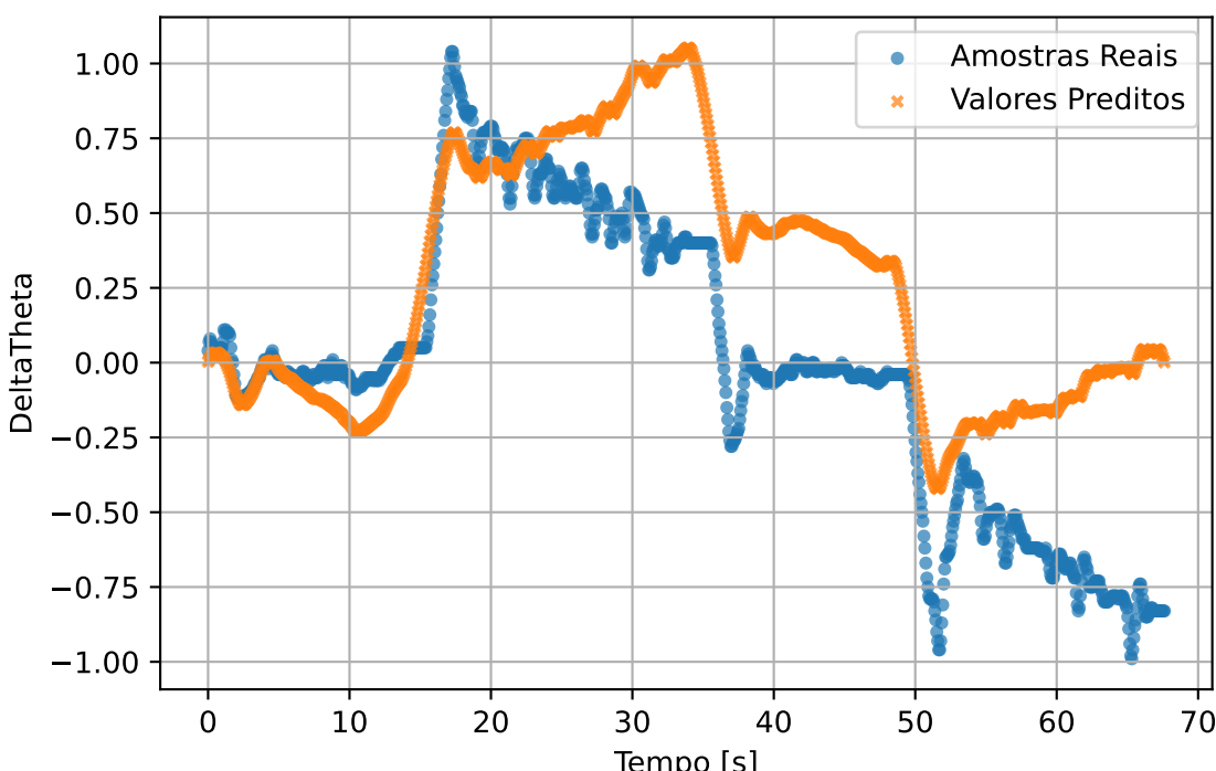
train2 - DeltaTheta
