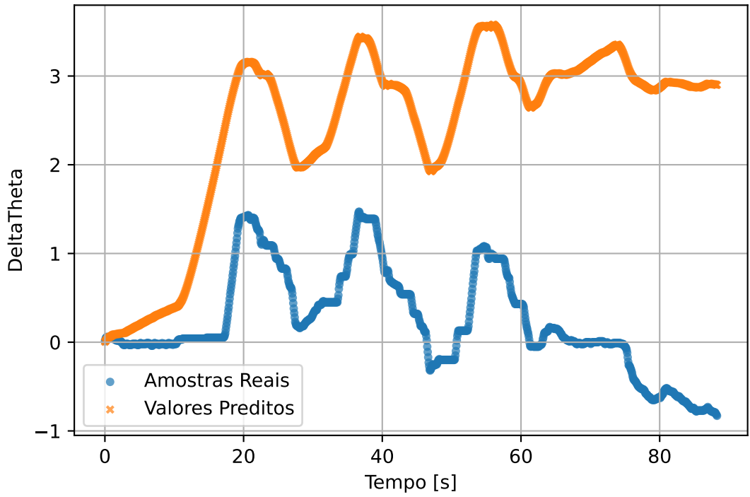
val - DeltaTheta
