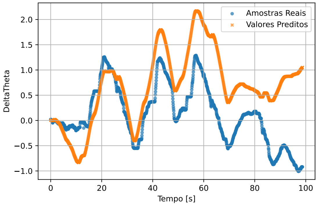
val - DeltaTheta
