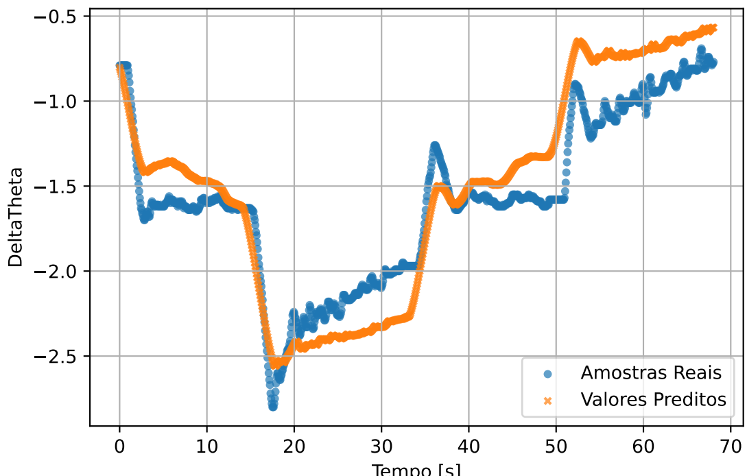
test3 - DeltaTheta
