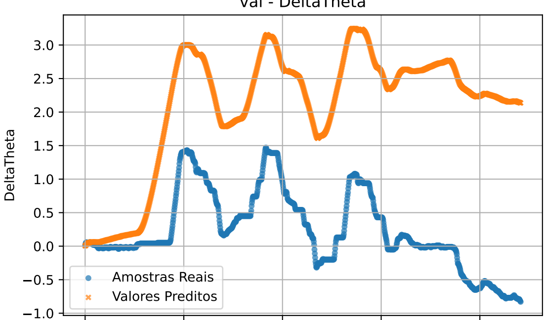
val - DeltaTheta
