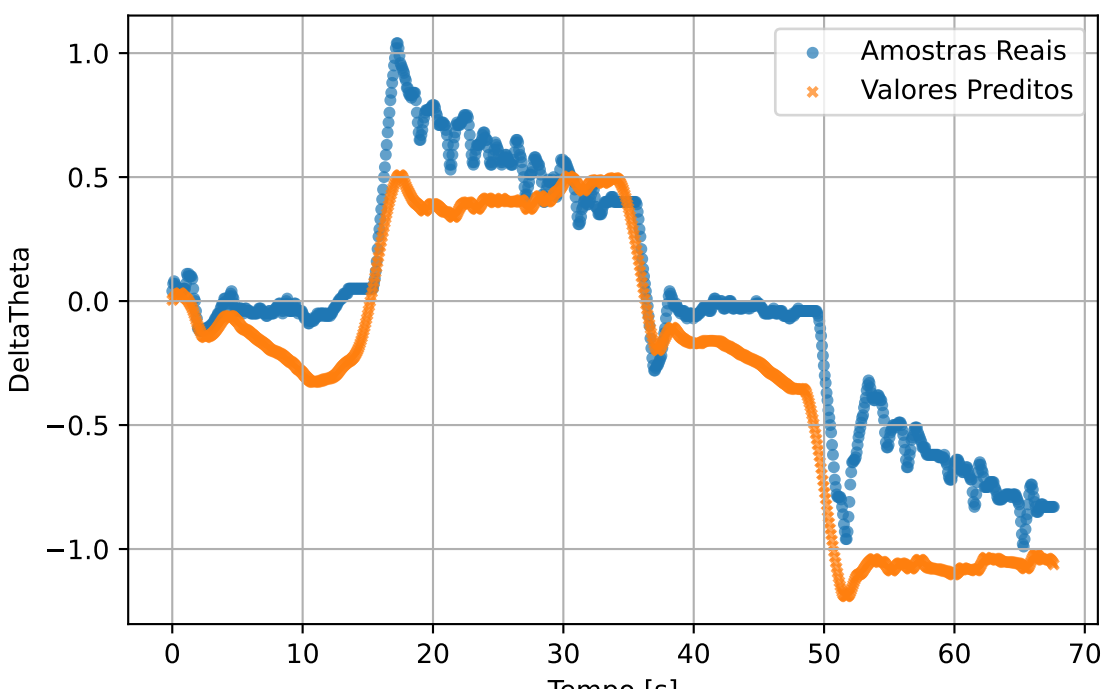
train2 - DeltaTheta
