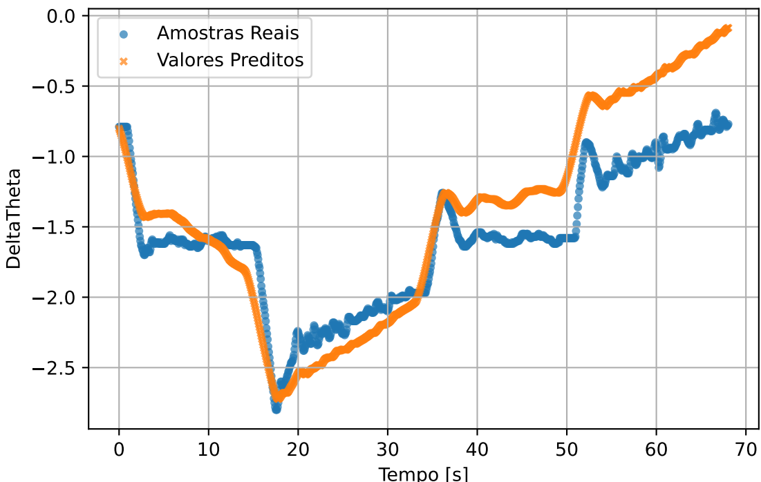
test3 - DeltaTheta
