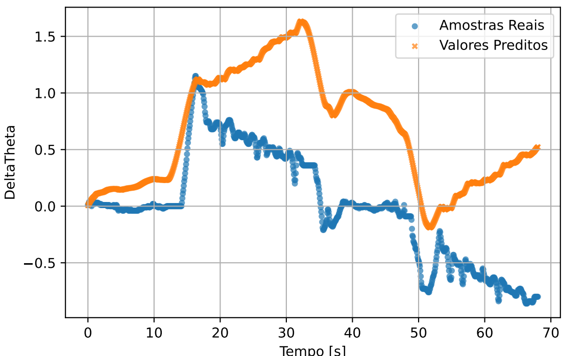
test2 - DeltaTheta
