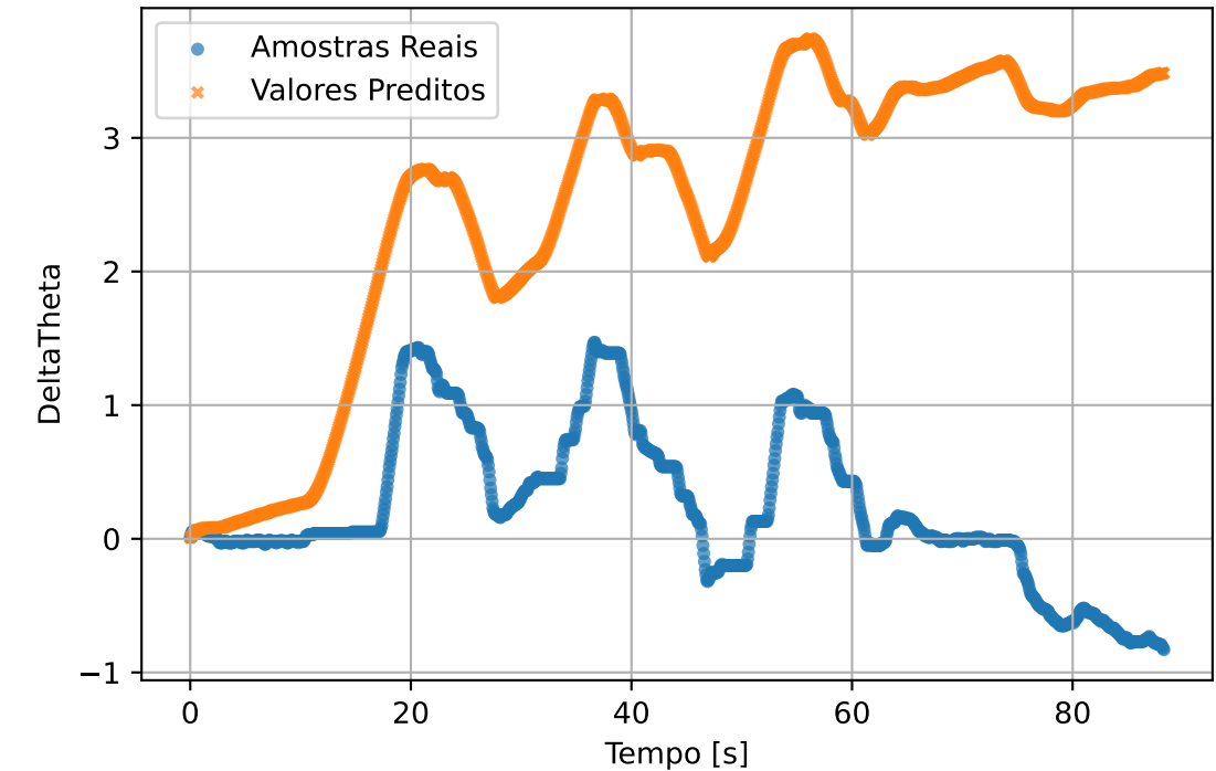
val - DeltaTheta
