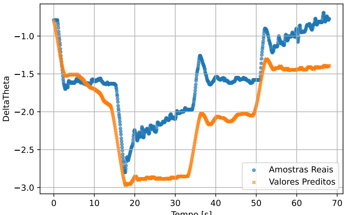
test3 - DeltaTheta
