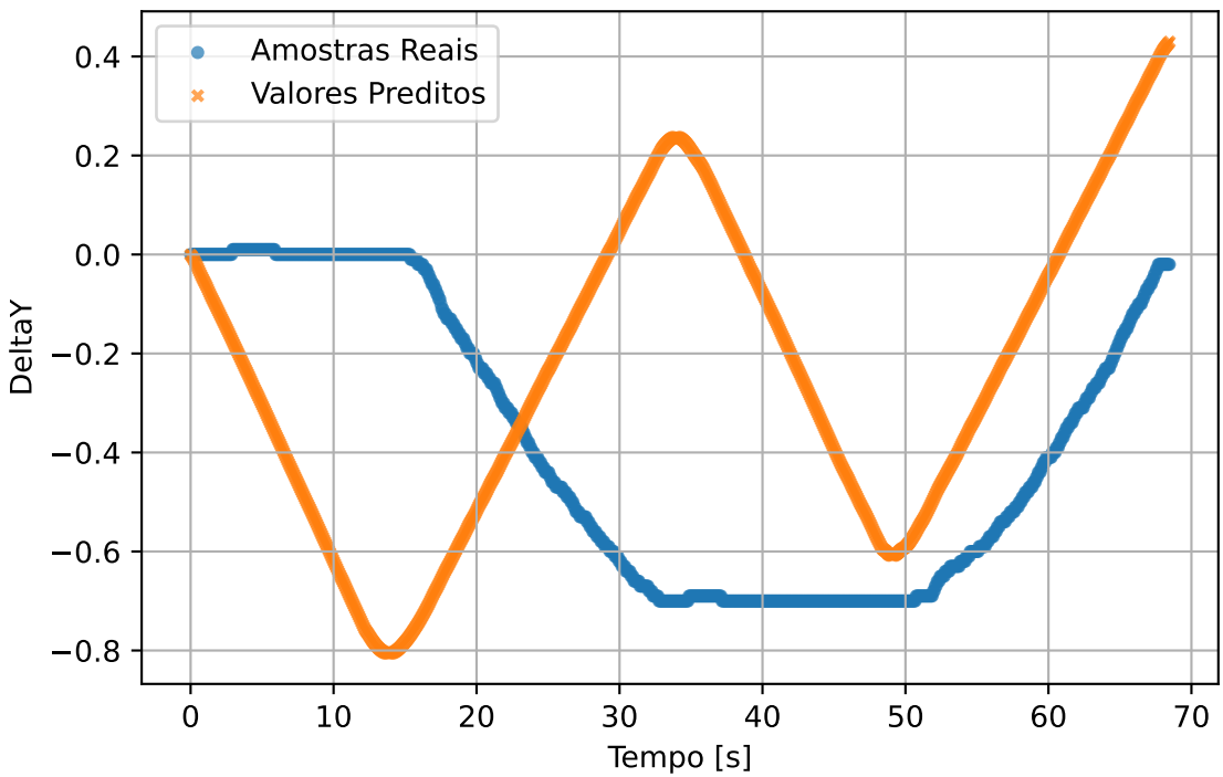
test2 - DeltaY
