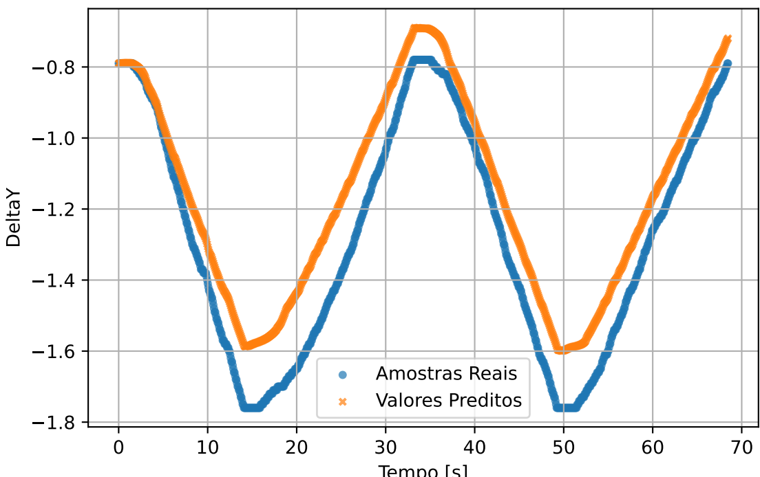
test3 - DeltaY
