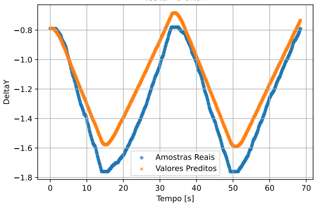
test3 - DeltaY
