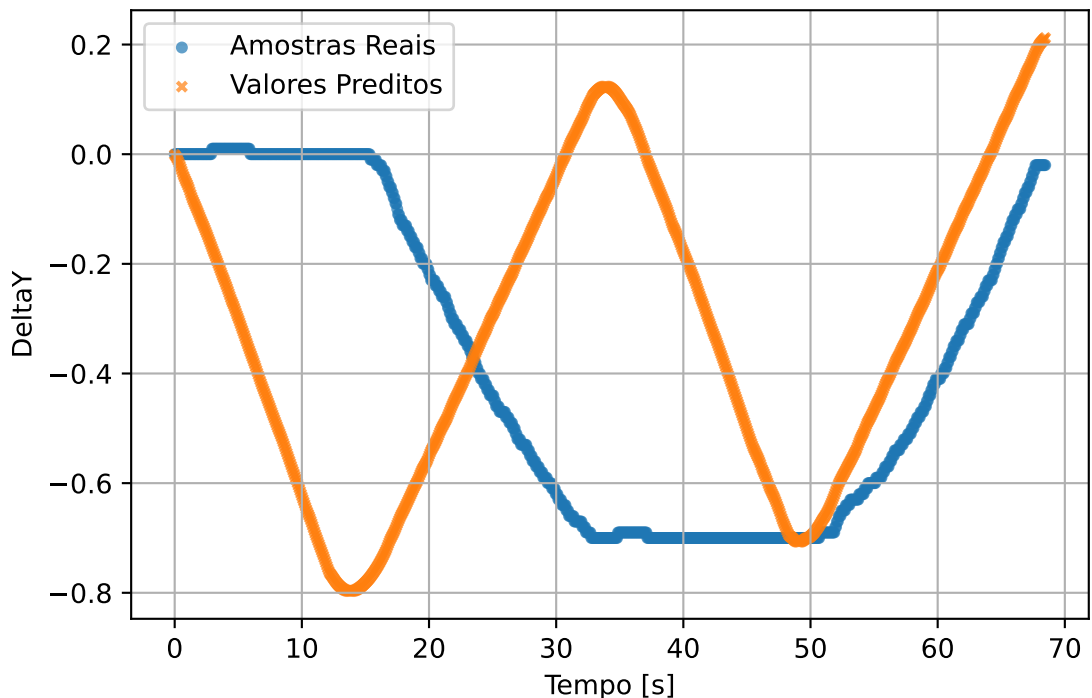
test2 - DeltaY
