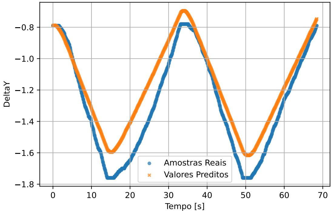
test3 - DeltaY
