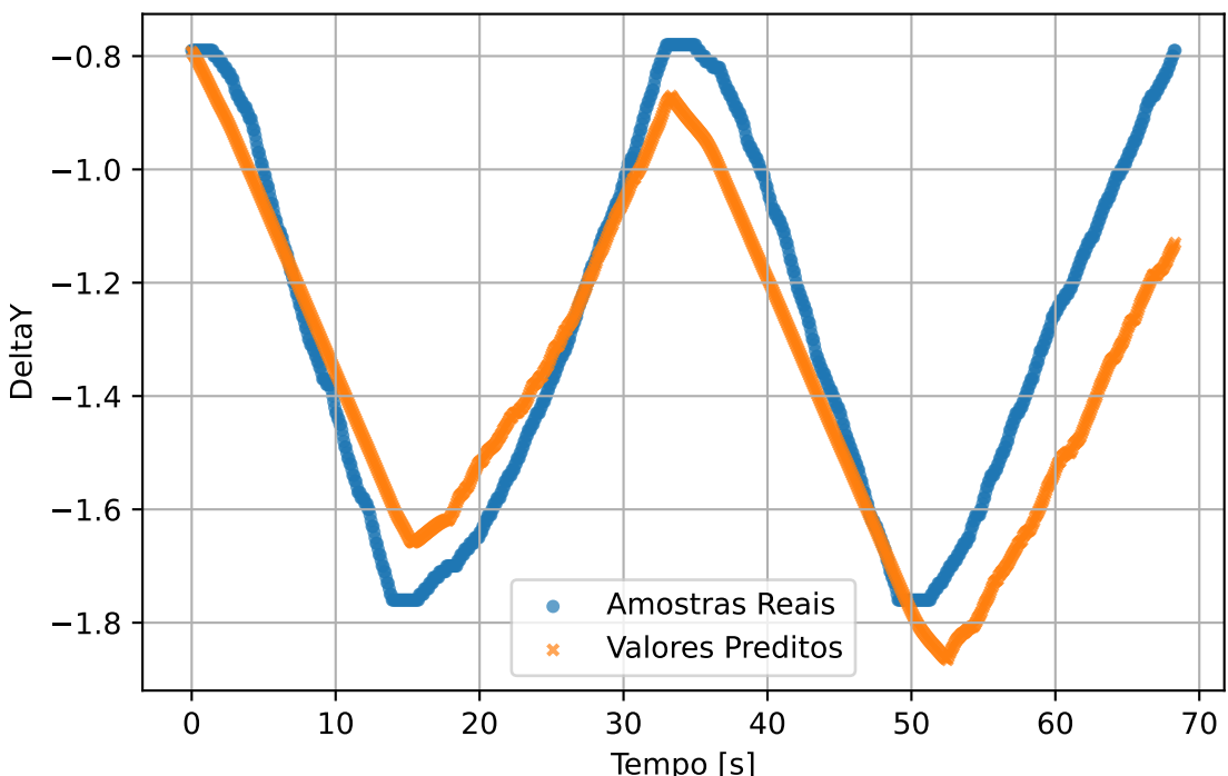
test3 - DeltaY
