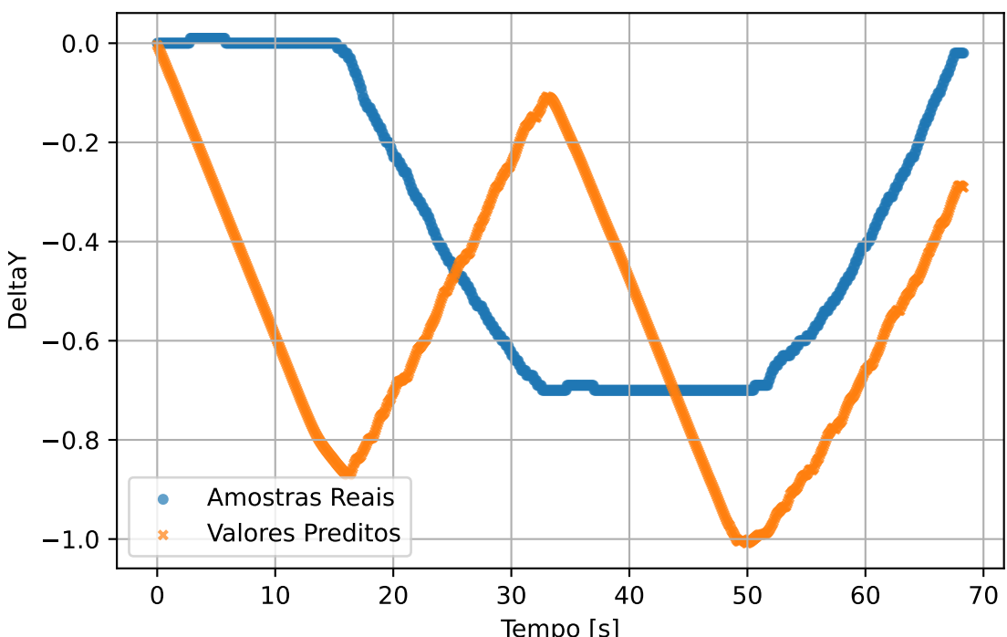
test2 - DeltaY
