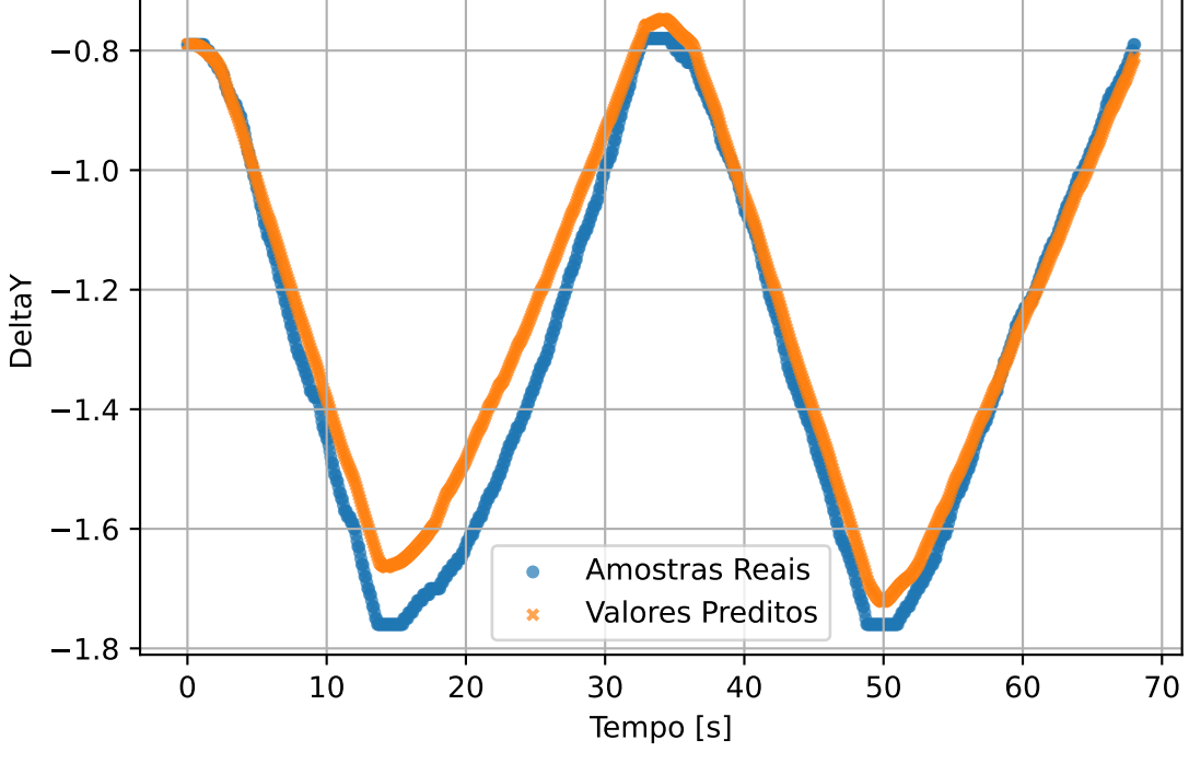
test3 - DeltaY
