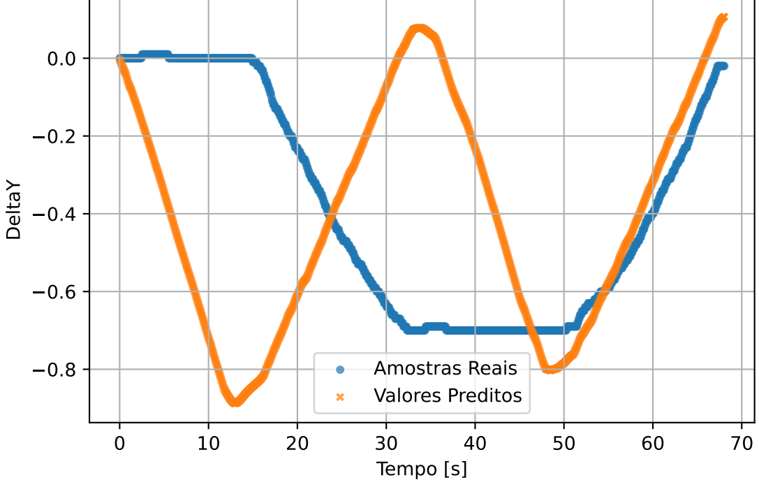
test2 - DeltaY
