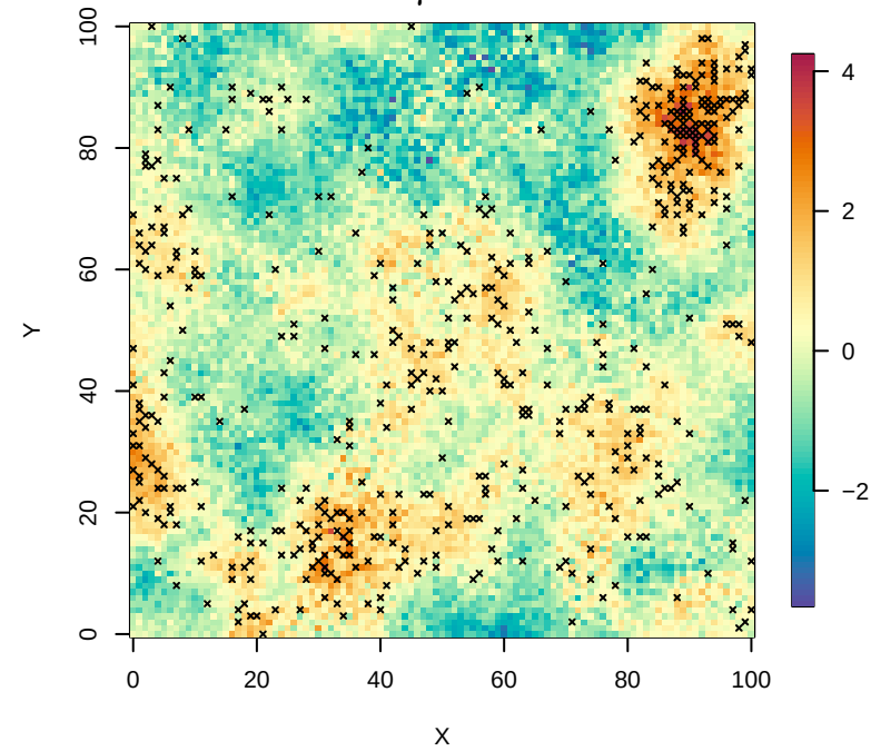
Muestreo preferencial fuerte
