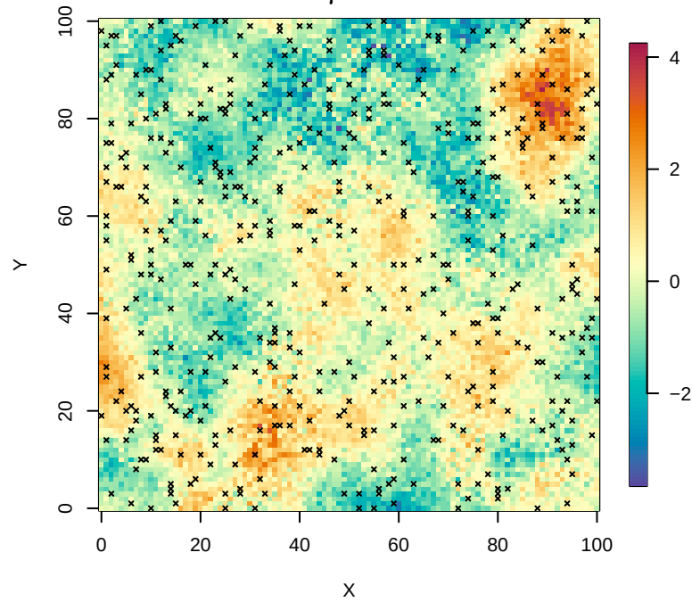
Muestreo aleatorio simple
