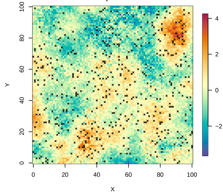
Muestreo preferencial moderado
