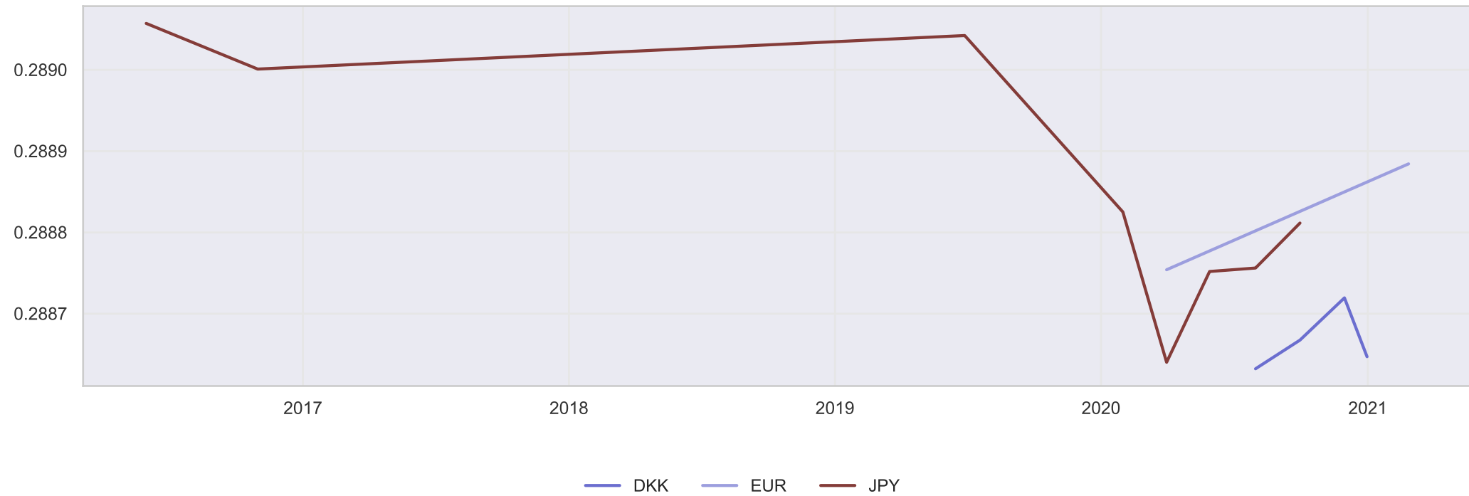
Drift \mu_3(z)
