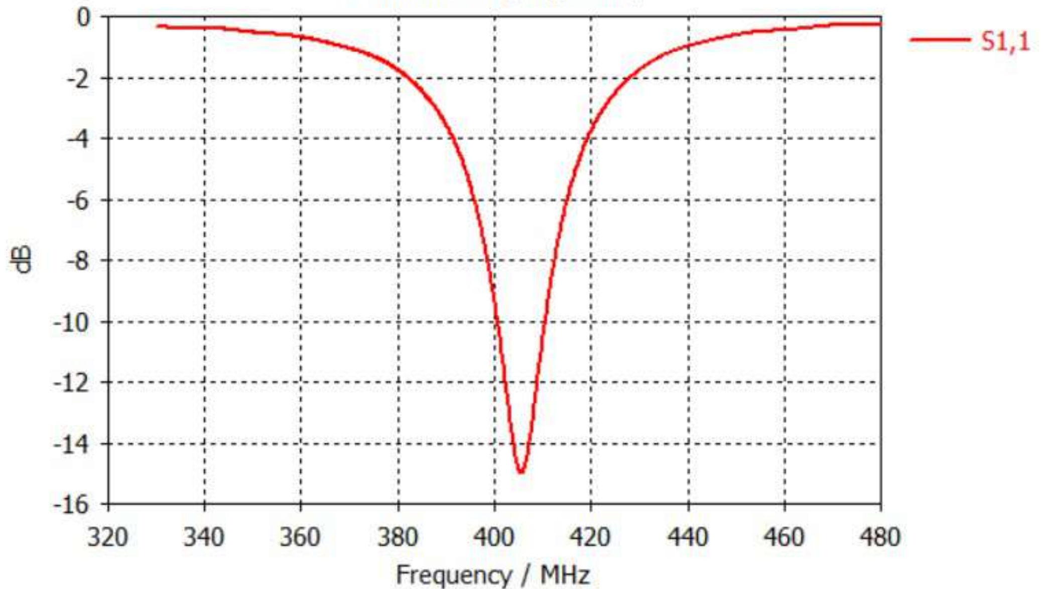
S-Parameters [Magnitude]
