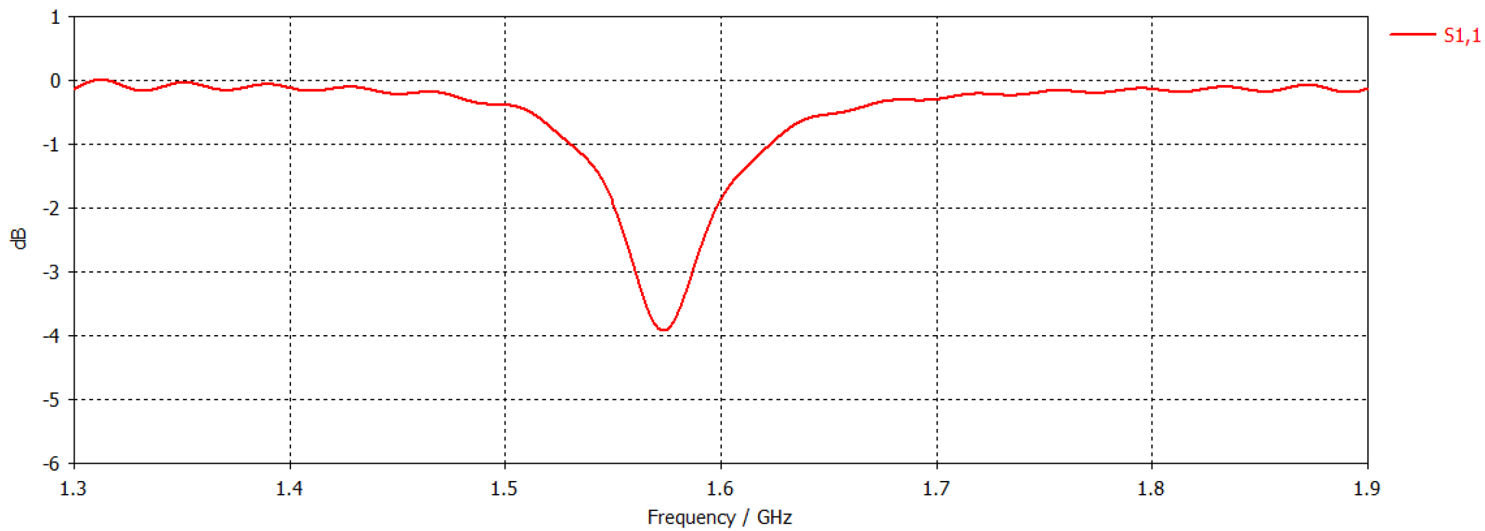
S-Parameters [Magnitude]
