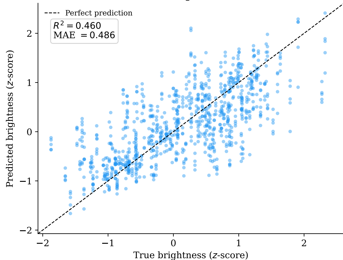
ImageNet
