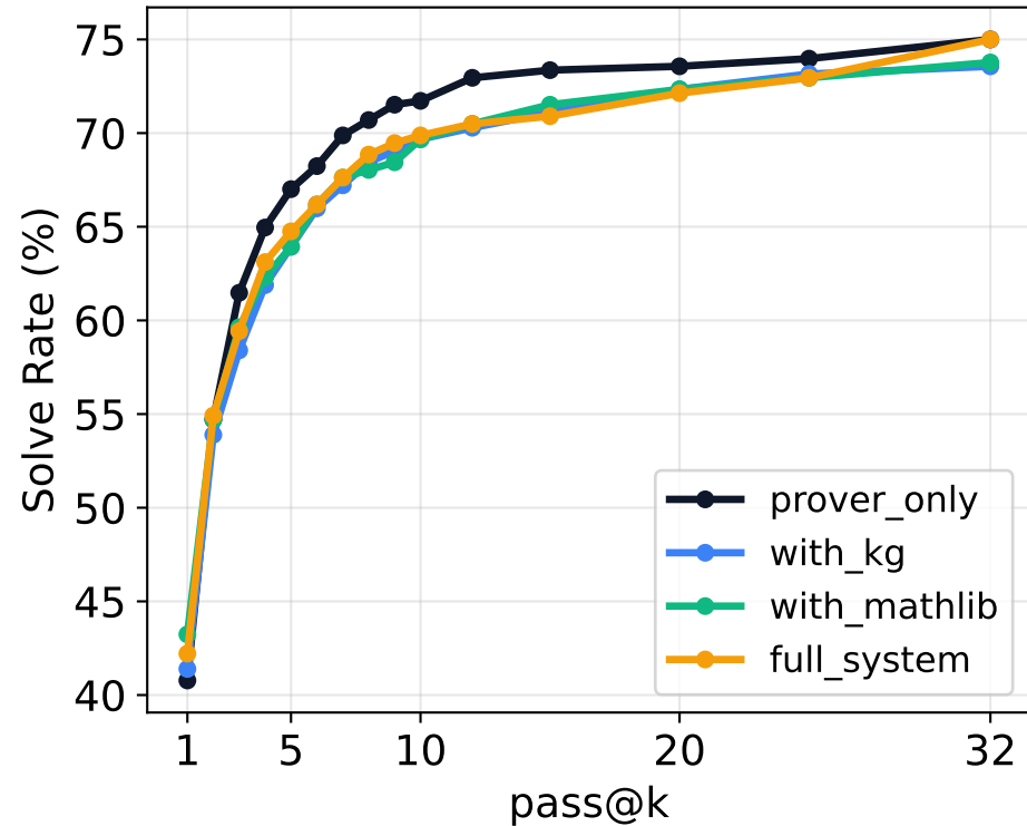
miniF2F
