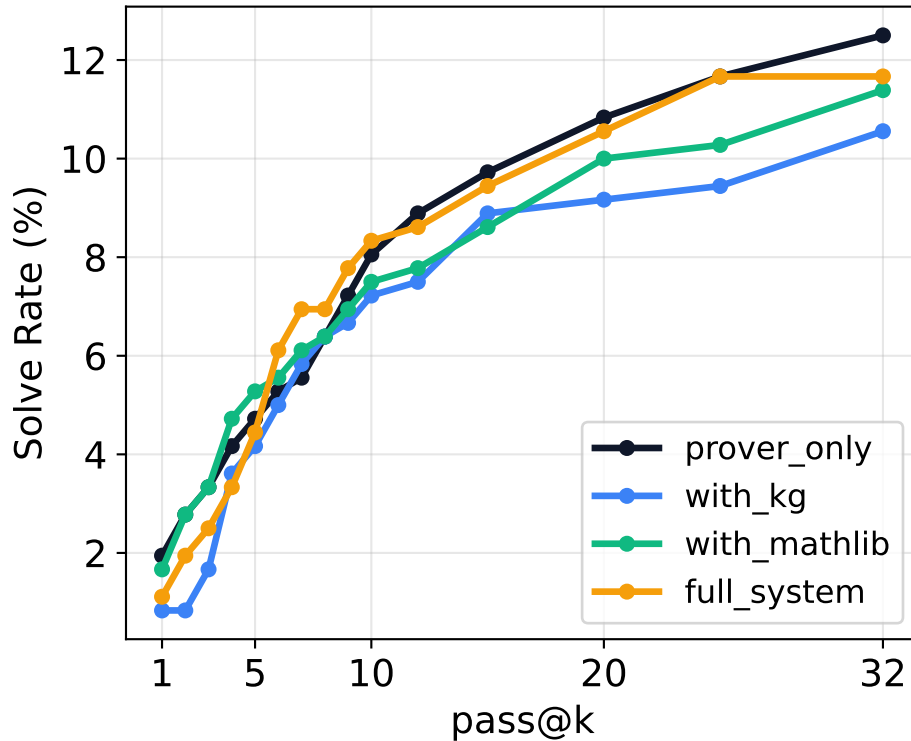
MathOlympiadBench
