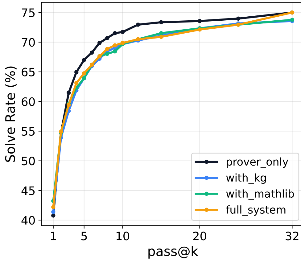
miniF2F (488)
