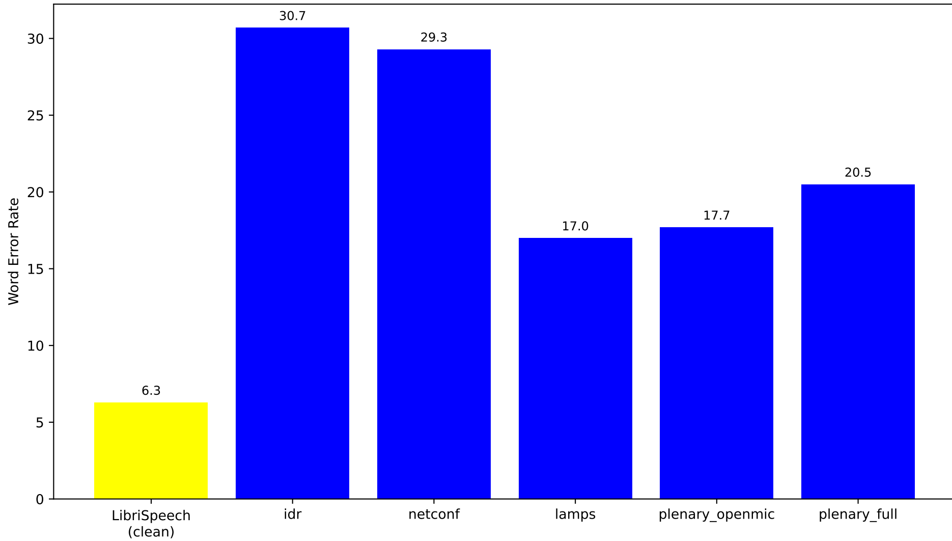
LibriSpeech Base Benchmark vs Base IETF Source
