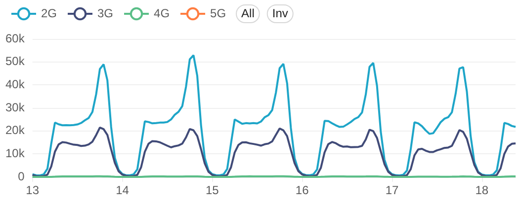
Voice Traffic (Erlangs)
