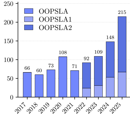
OOPSLA
