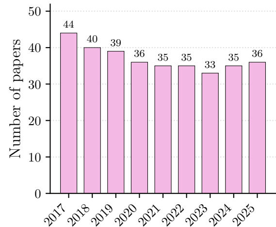
ICFP
