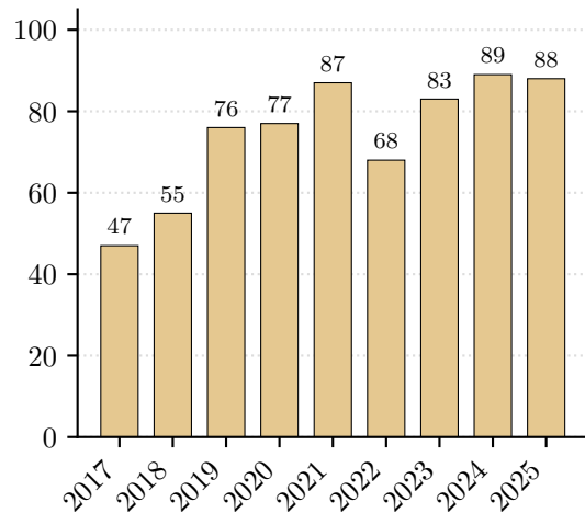
PLDI
