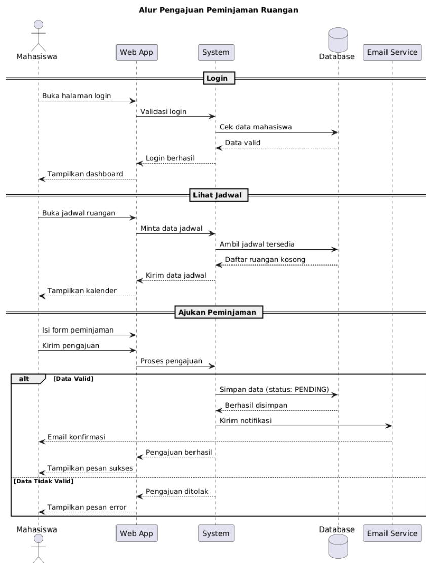
Gambar 3.6: Sequence Diagram Pengajuan Peminjaman
