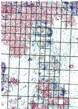
Xenium (165 tiles)
