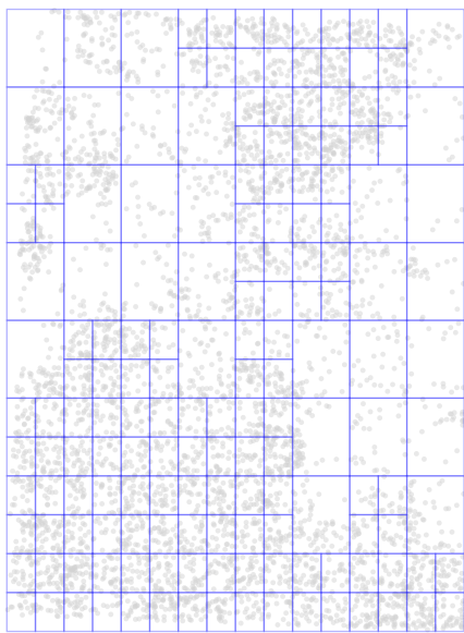
Xenium (166 tiles)
